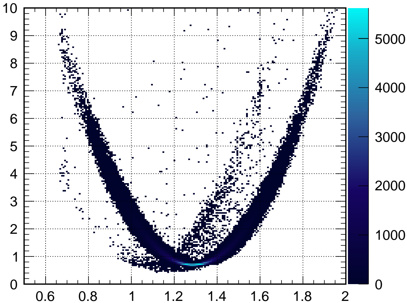
LogL_sample_0:xsec_28
