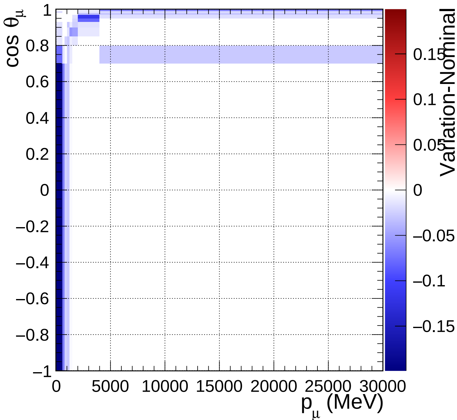
FGD2_anti-numuCC_other_Q2_norm_6_0.82
