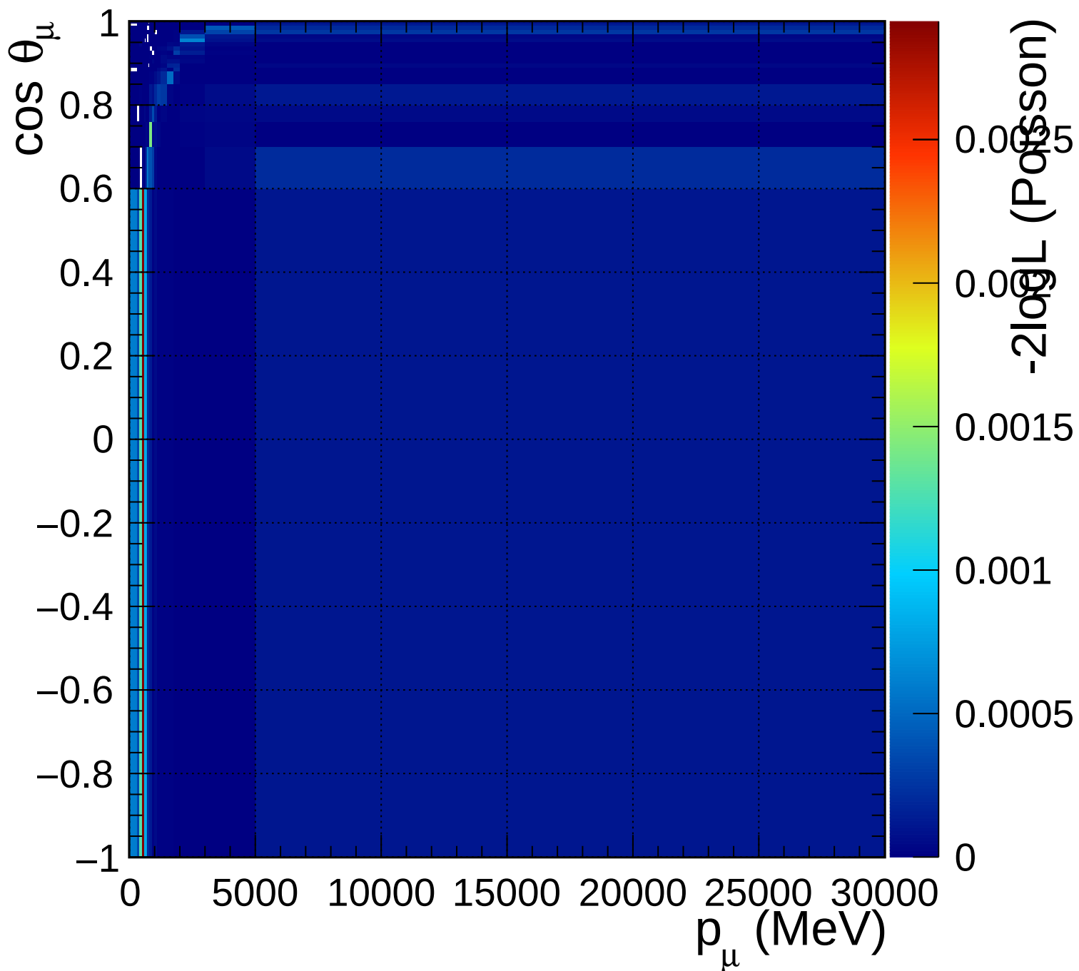
FGD2_numuCC_other_Q2_norm_6_1.18
