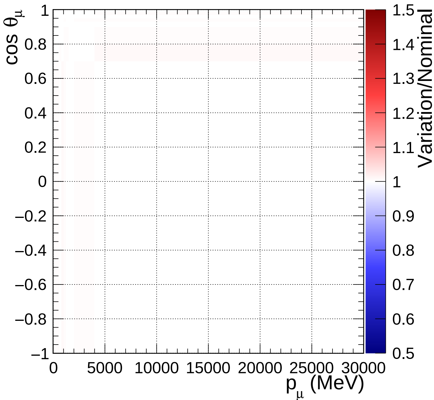
FGD1_anti-numuCC_other_Q2_norm_6_1.18
