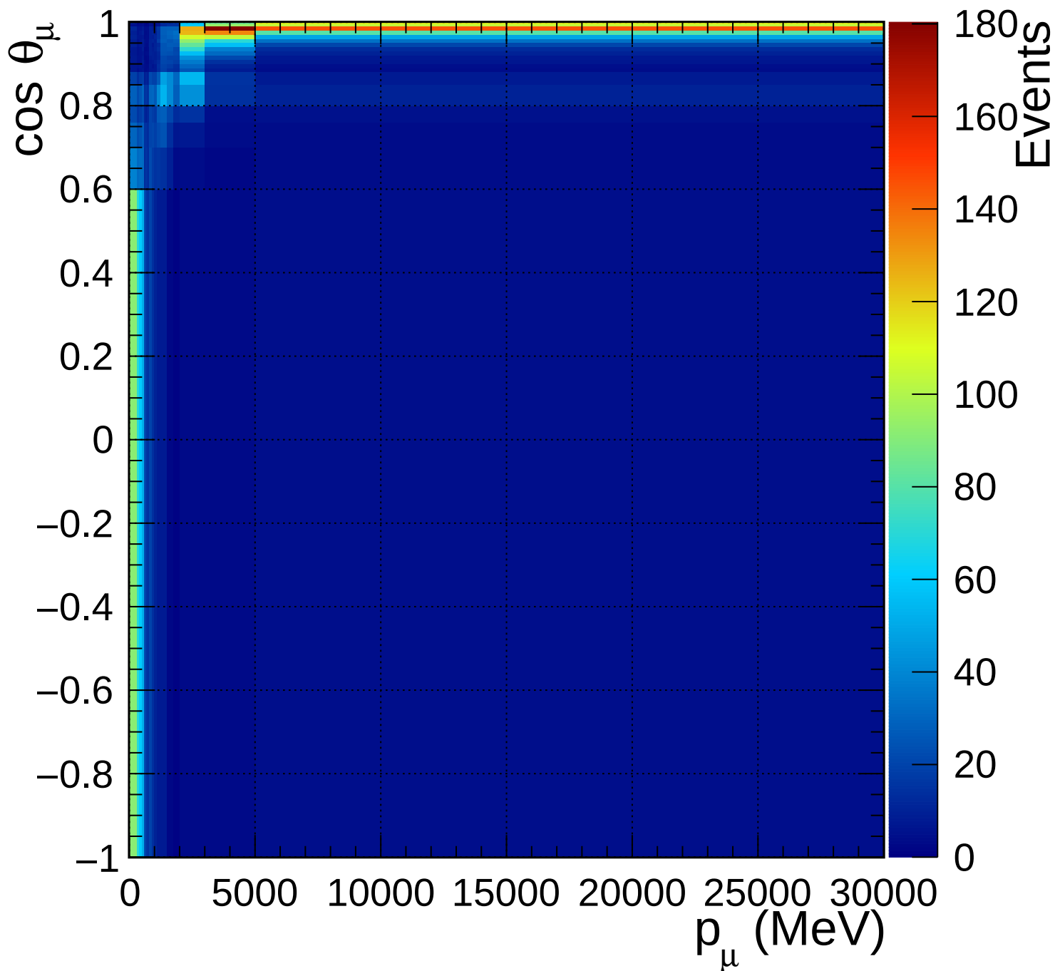
FGD2_numuCC_other_Q2_norm_7_1
