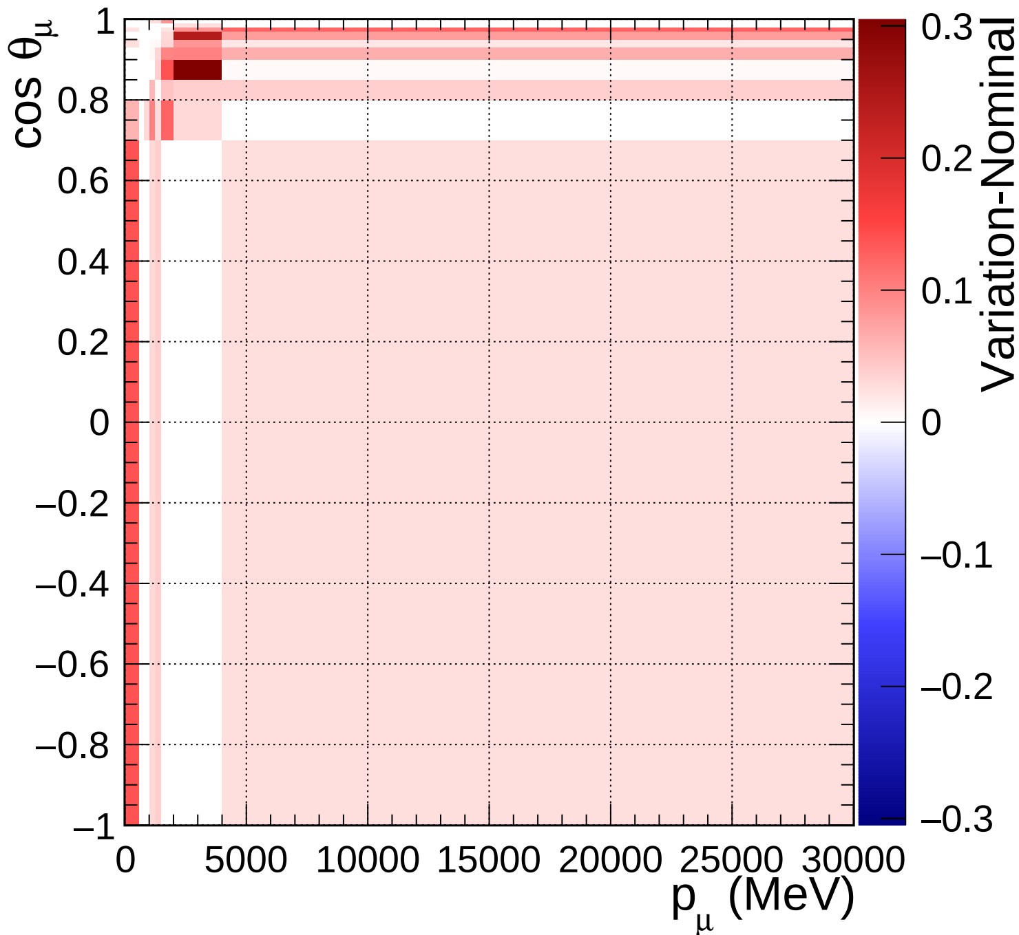
FGD2_anti-numuCC_other_Q2_norm_7_1.4
