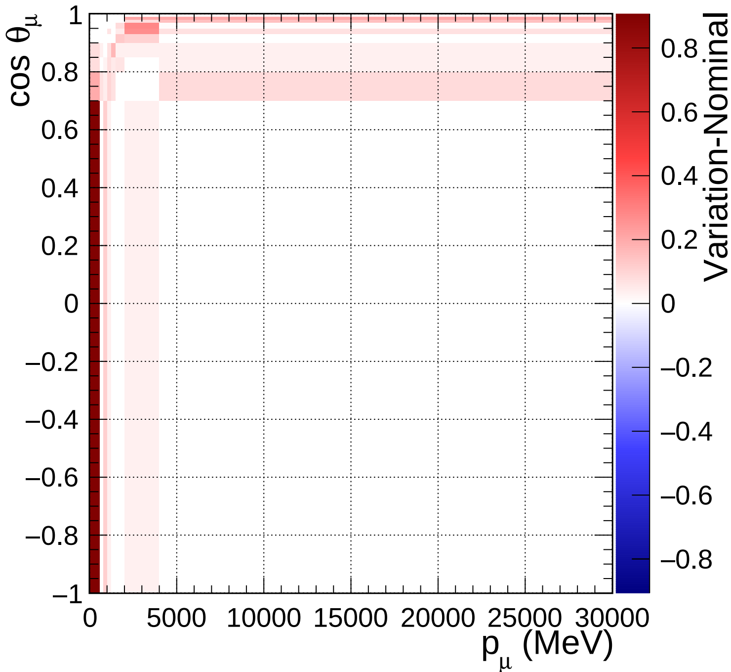
FGD1_anti-numuCC_other_Q2_norm_6_1.54
