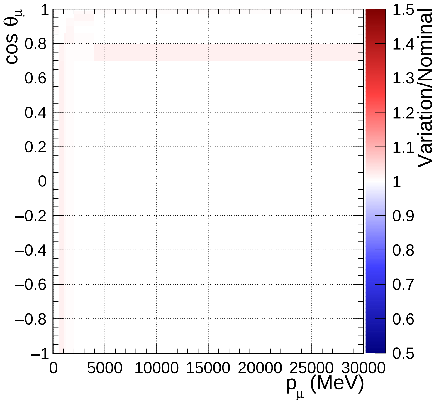
FGD1_NuMuBkg_CCother_in_AntiNu_Mode_Q2_norm_6_1.54
