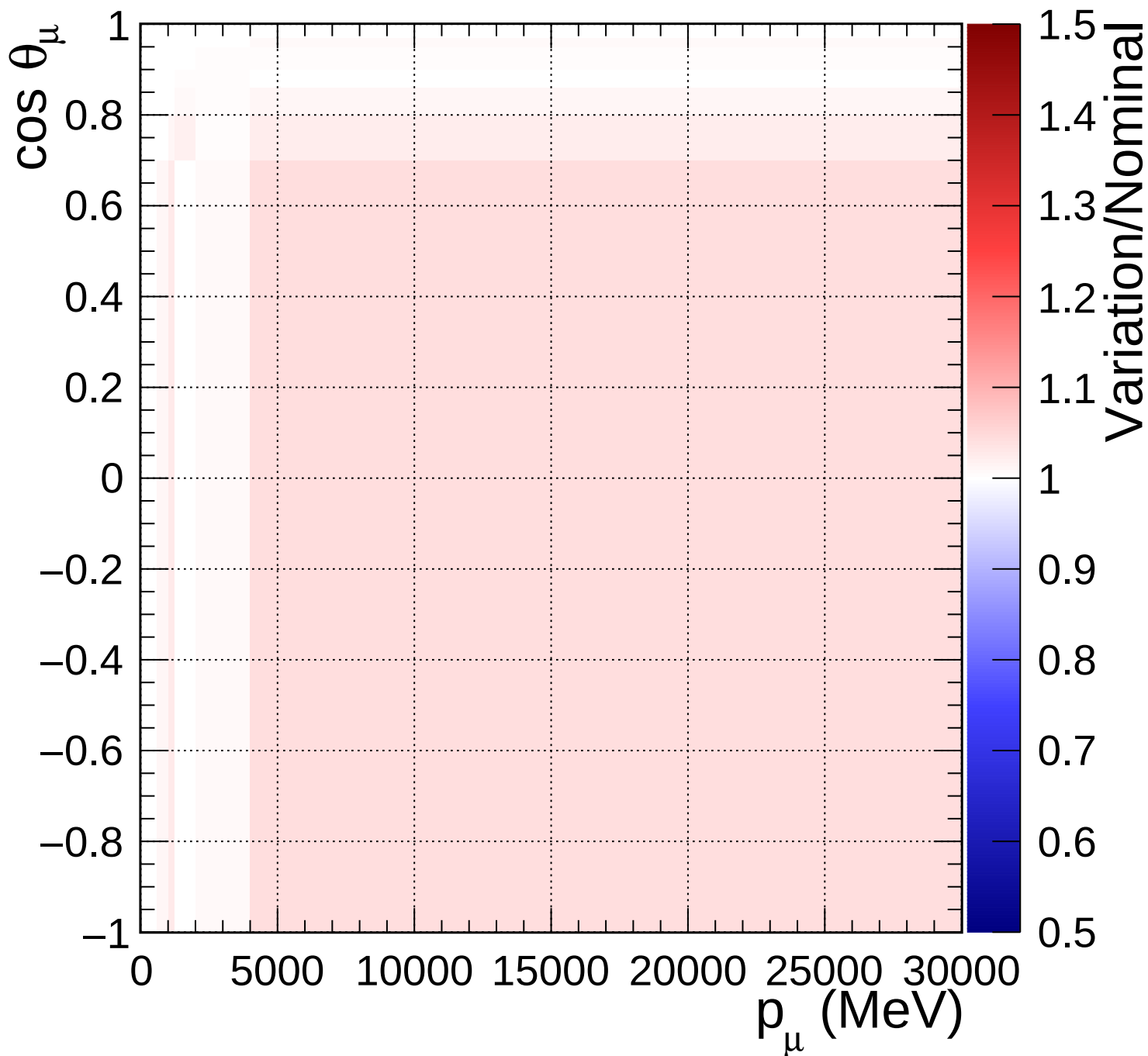
FGD1_NuMuBkg_CCoher_in_AntiNu_Mode_Q2_norm_7_1.4
