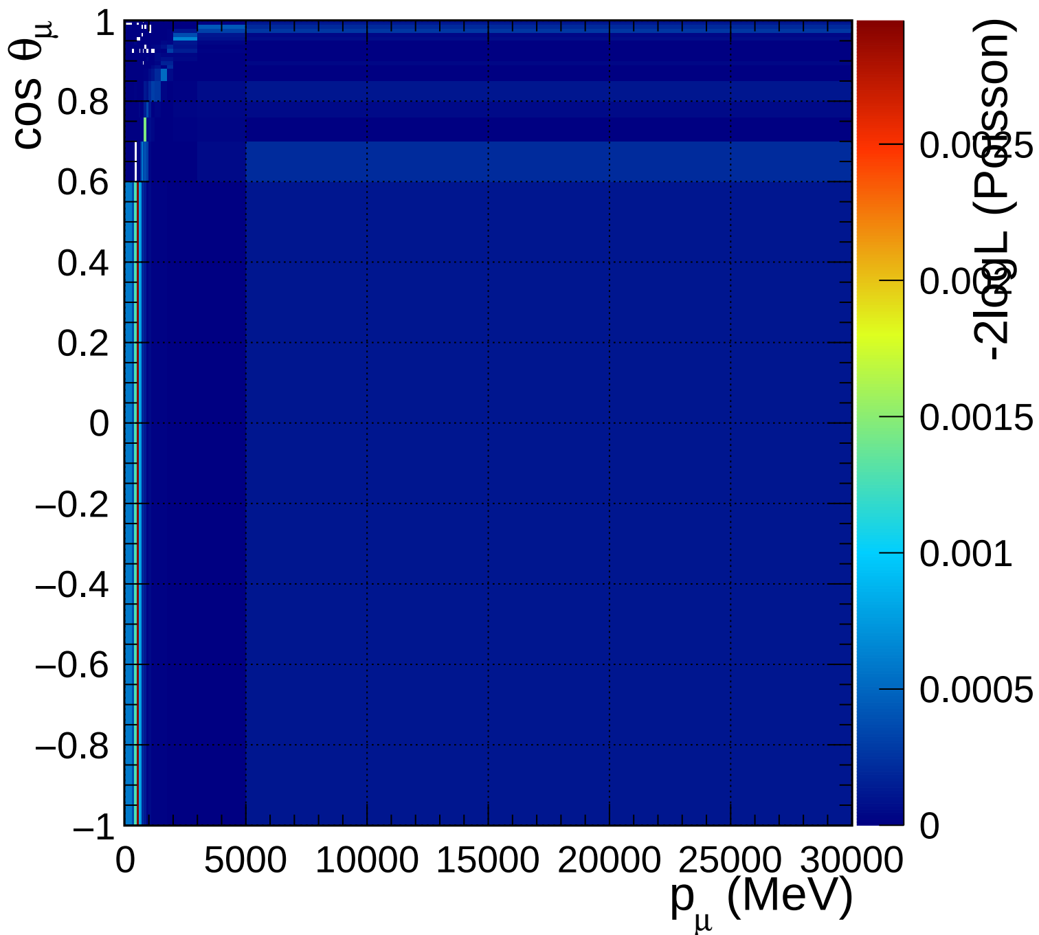
FGD2_numuCC_other_Q2_norm_6_0.82
