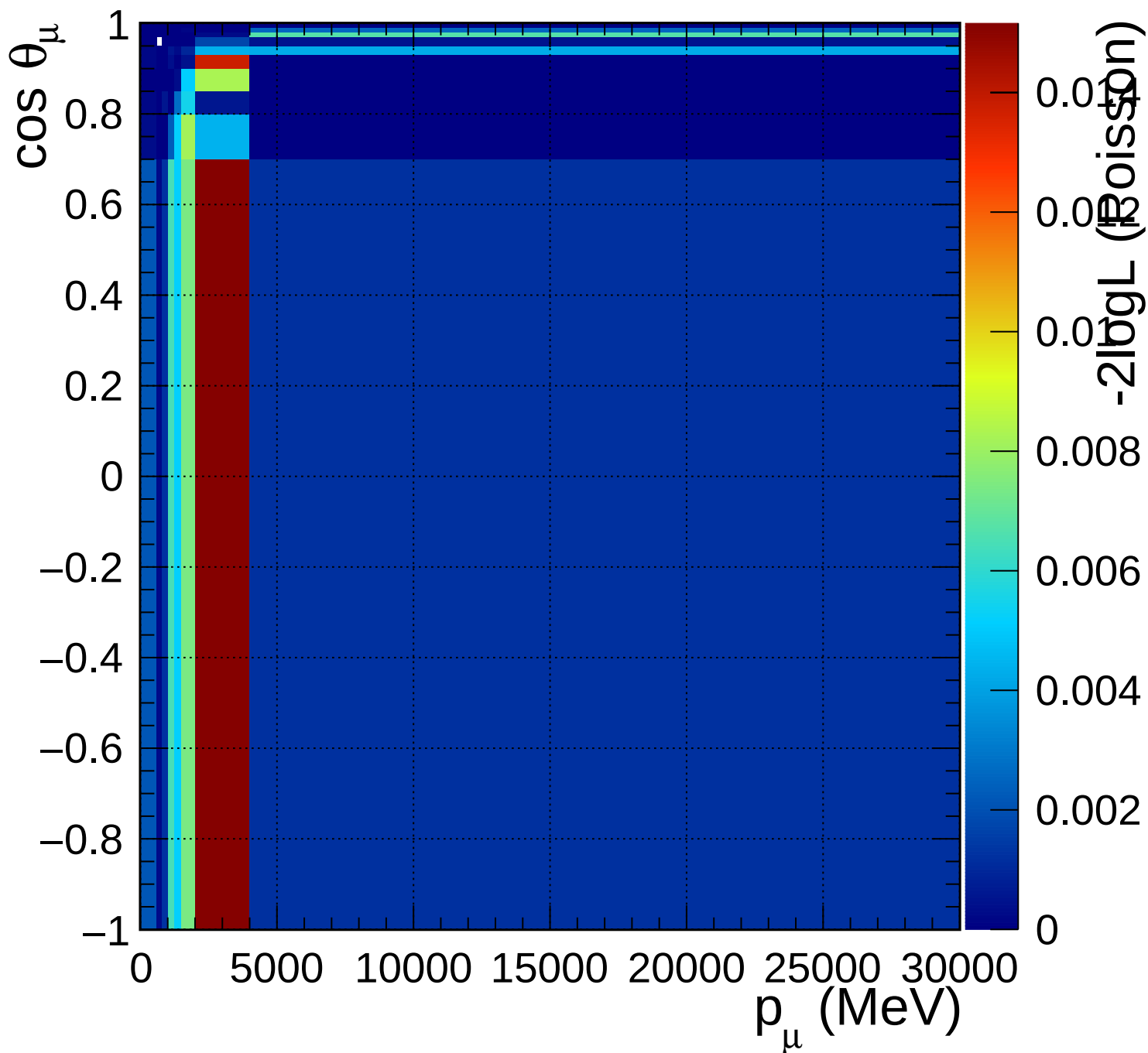
FGD1_anti-numuCC_other_Q2_norm_7_2.2
