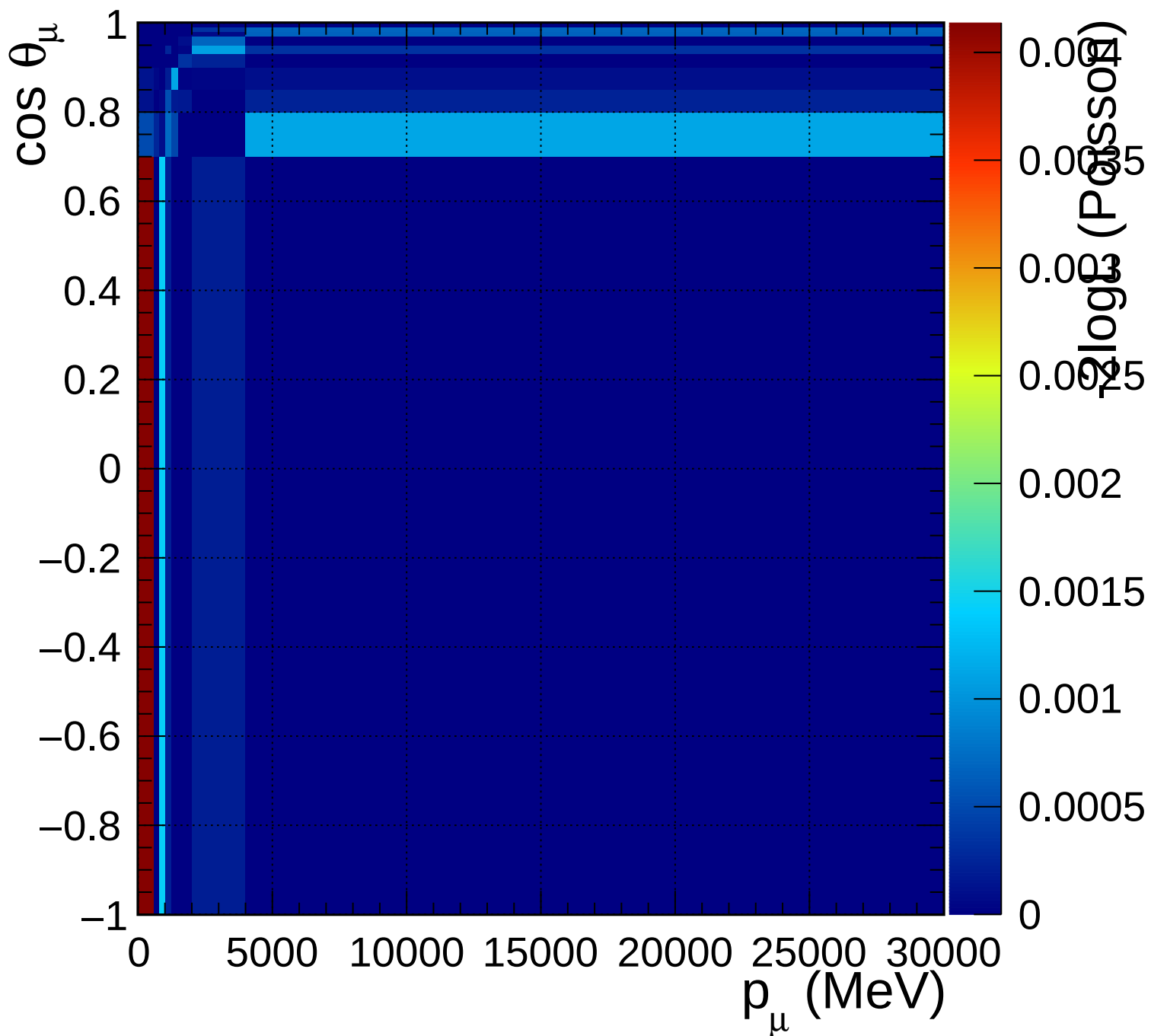
FGD1_anti-numuCC_other_Q2_norm_6_1.54
