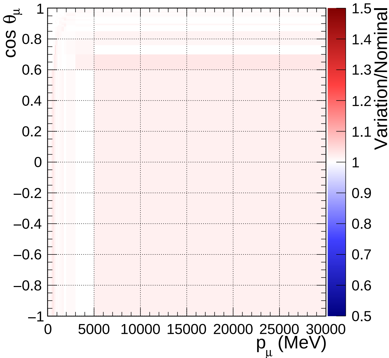
FGD2_numuCC_other_Q2_norm_6_1.54
