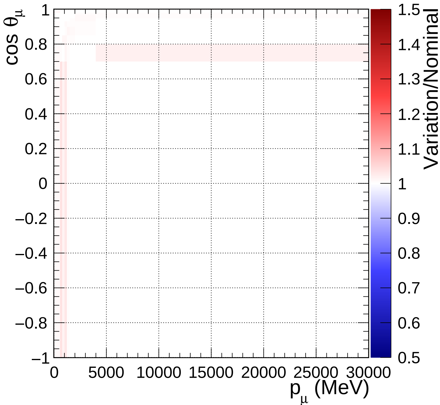
FGD2_anti-numuCC_other_Q2_norm_6_1.54
