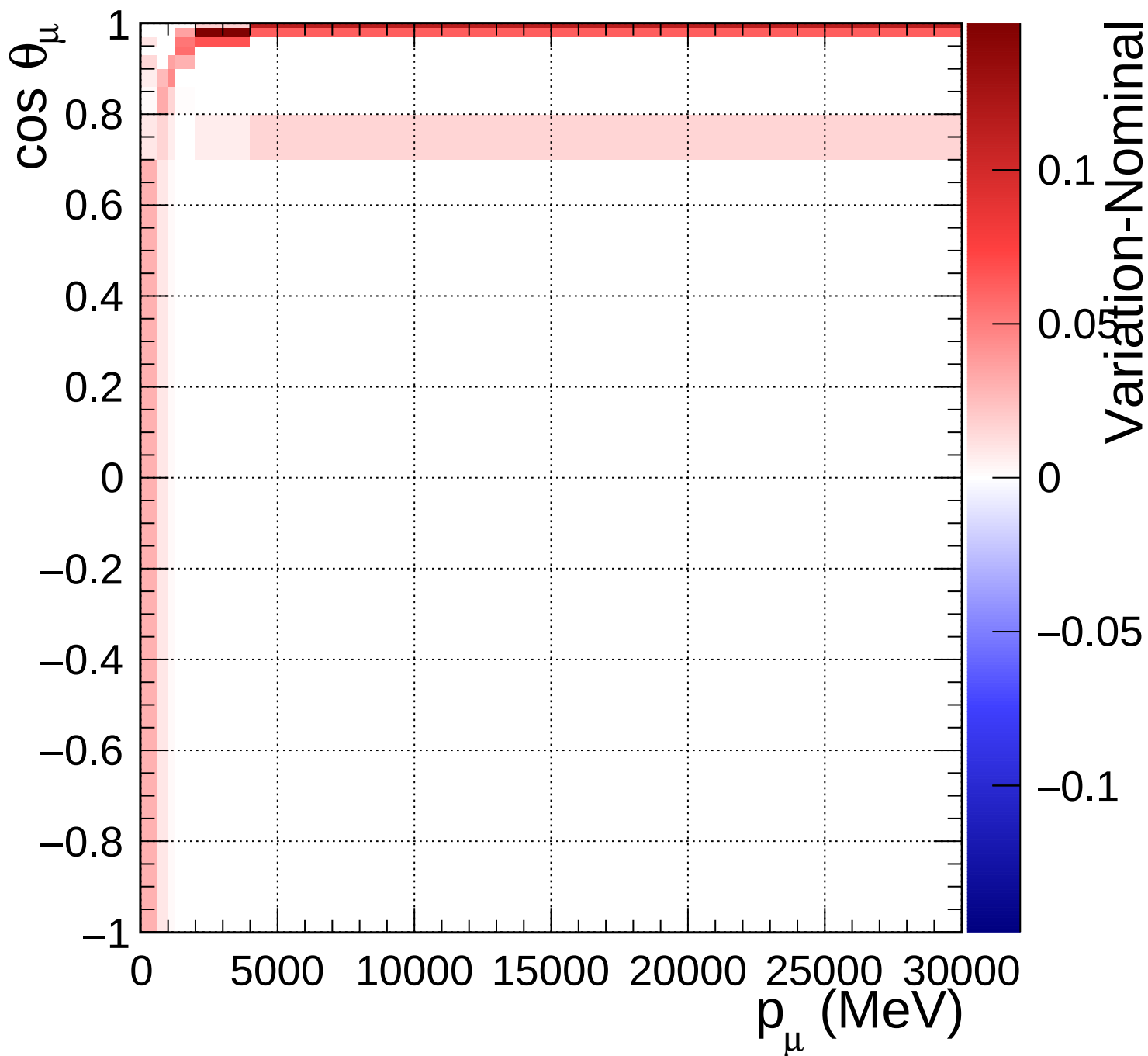
FGD1_NuMuBkg_CCoher_in_AntiNu_Mode_Q2_norm_5_1.11
