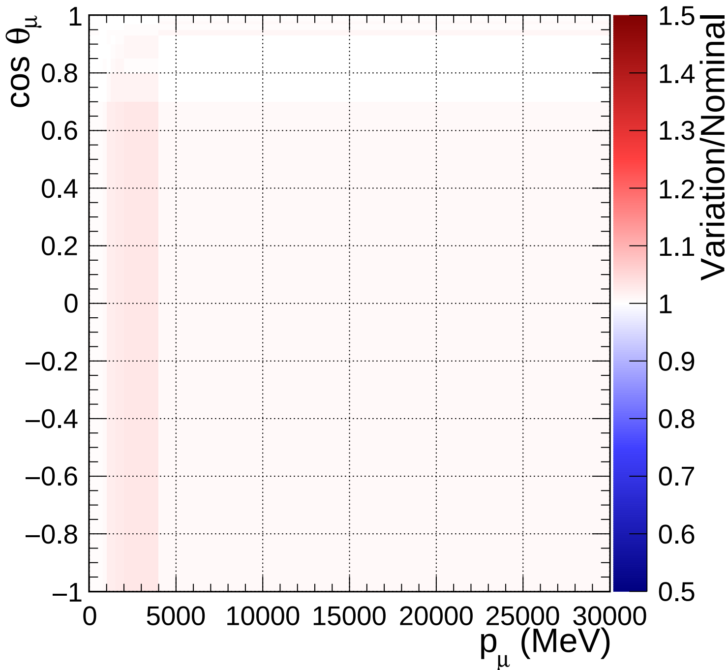
FGD1_anti-numuCC_other_Q2_norm_7_1.4
