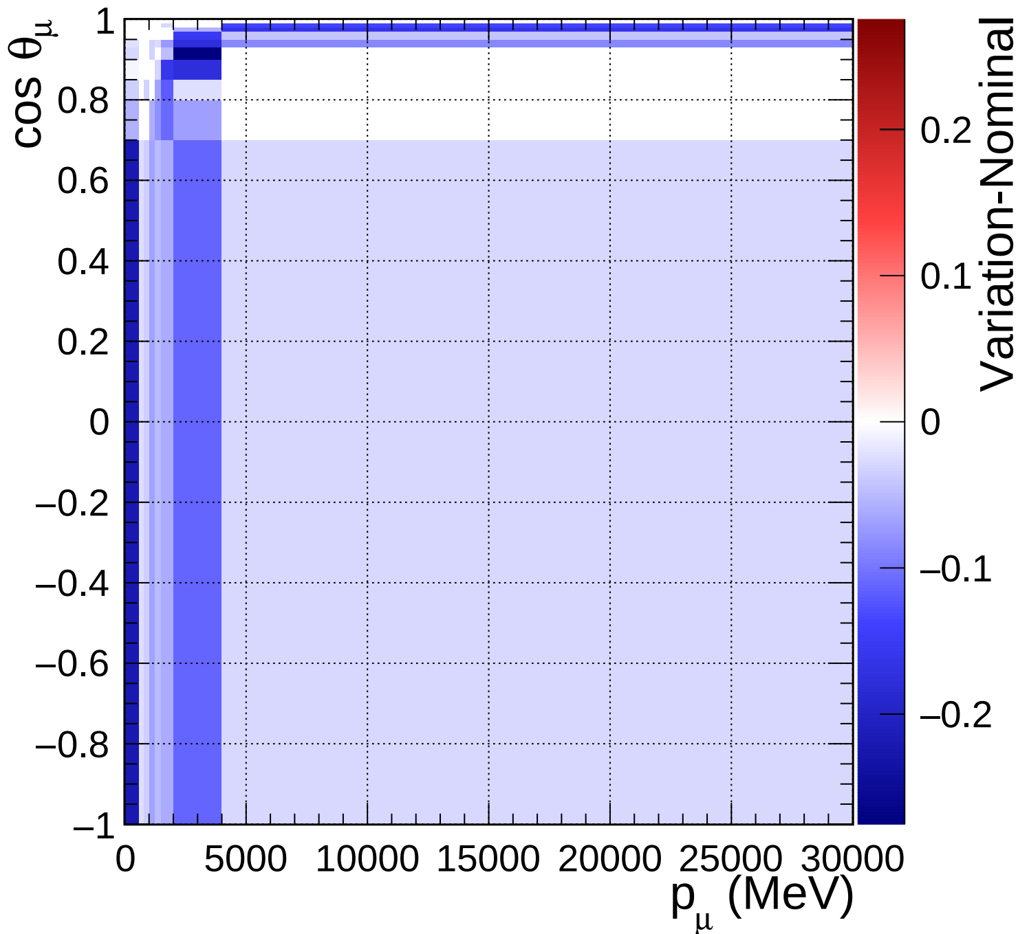
FGD1_anti-numuCC_other_Q2_norm_7_0.6
