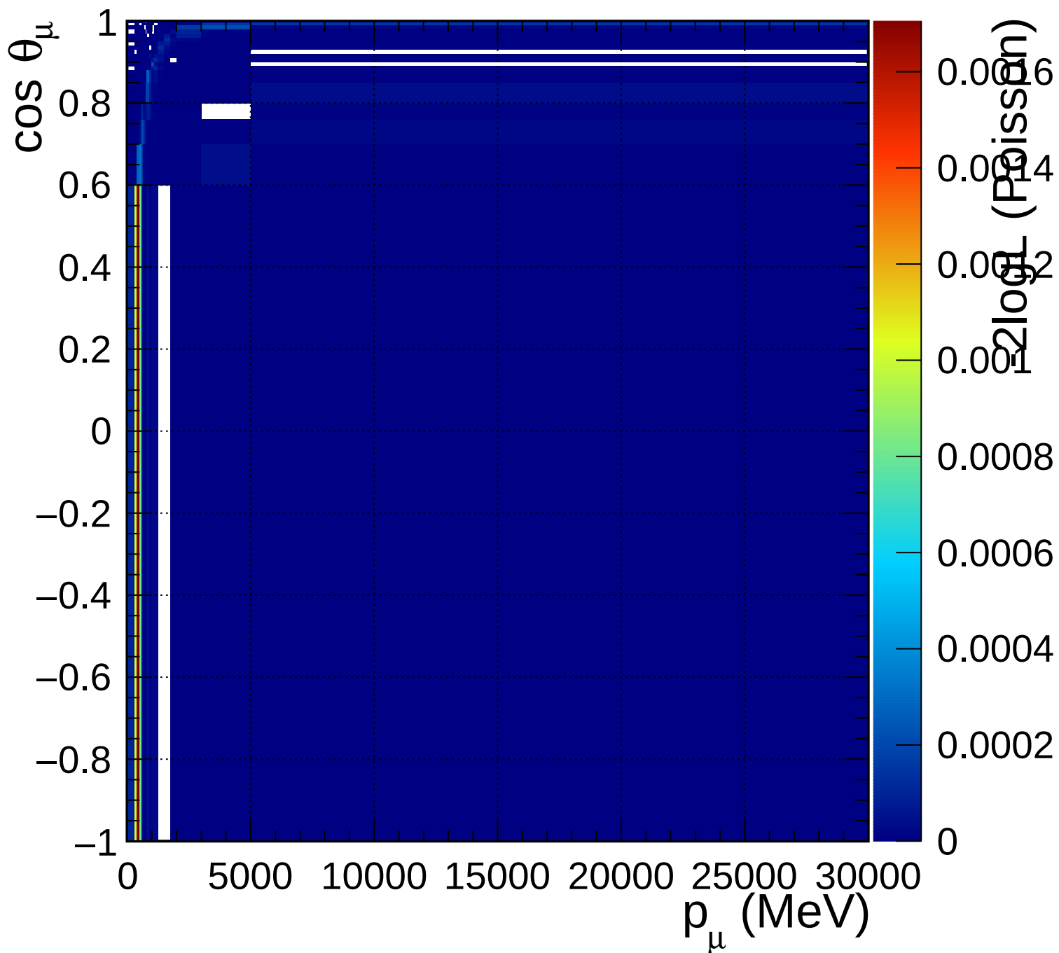
FGD2_numuCC_other_Q2_norm_5_0.89
