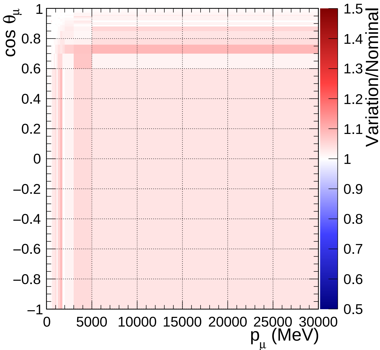
FGD2_numuCC_other_Q2_norm_7_2.2
