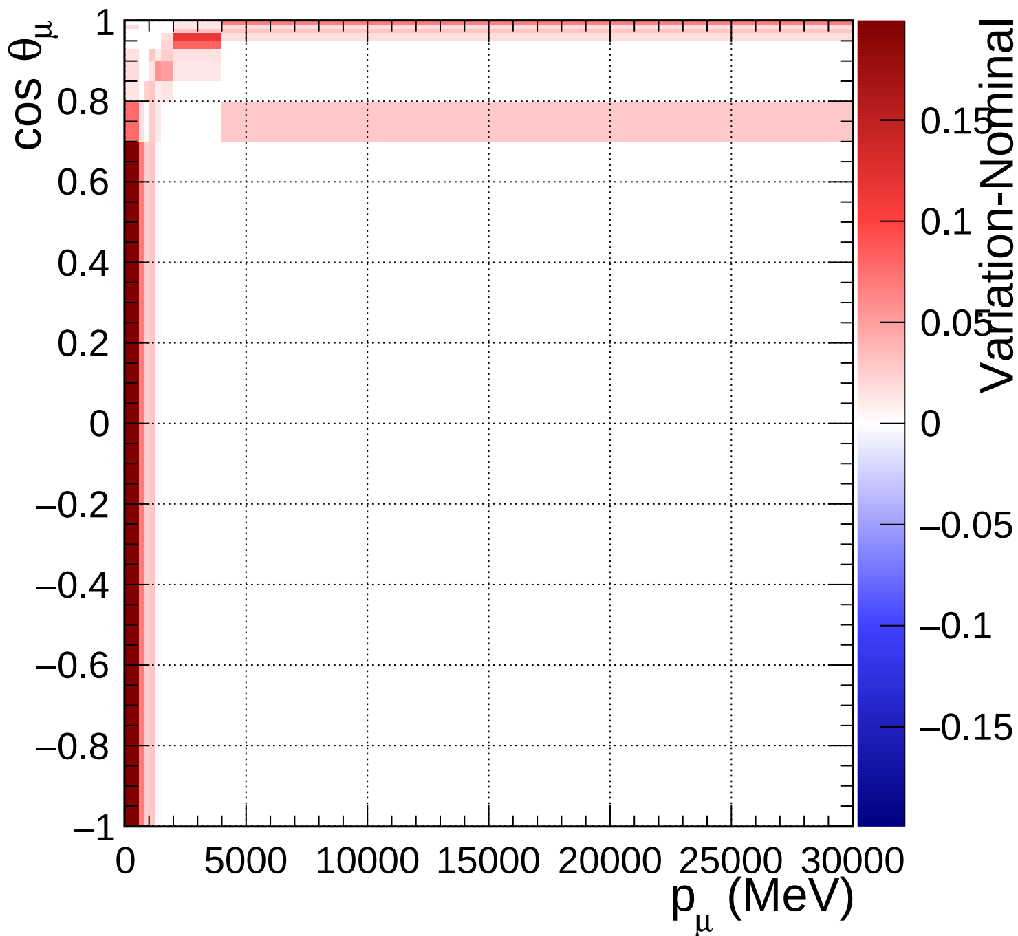
FGD2_anti-numuCC_other_Q2_norm_6_1.18
