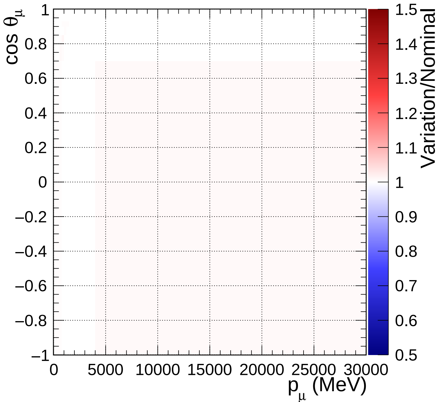
FGD2_anti-numuCC_other_Q2_norm_5_1.11
