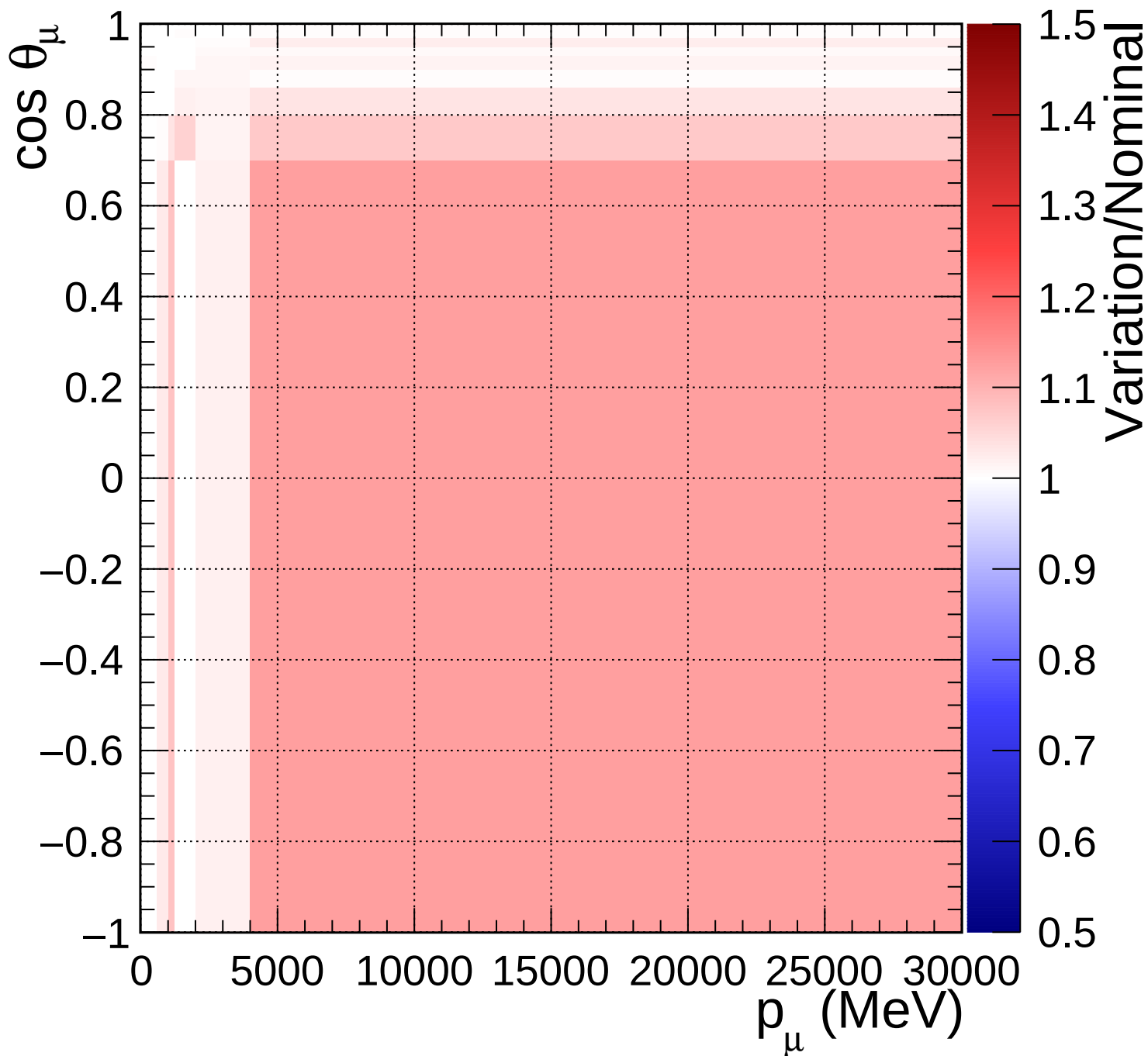
FGD1_NuMuBkg_CCoTher_in_AntiNu_Mode_Q2_norm_7_2.2
