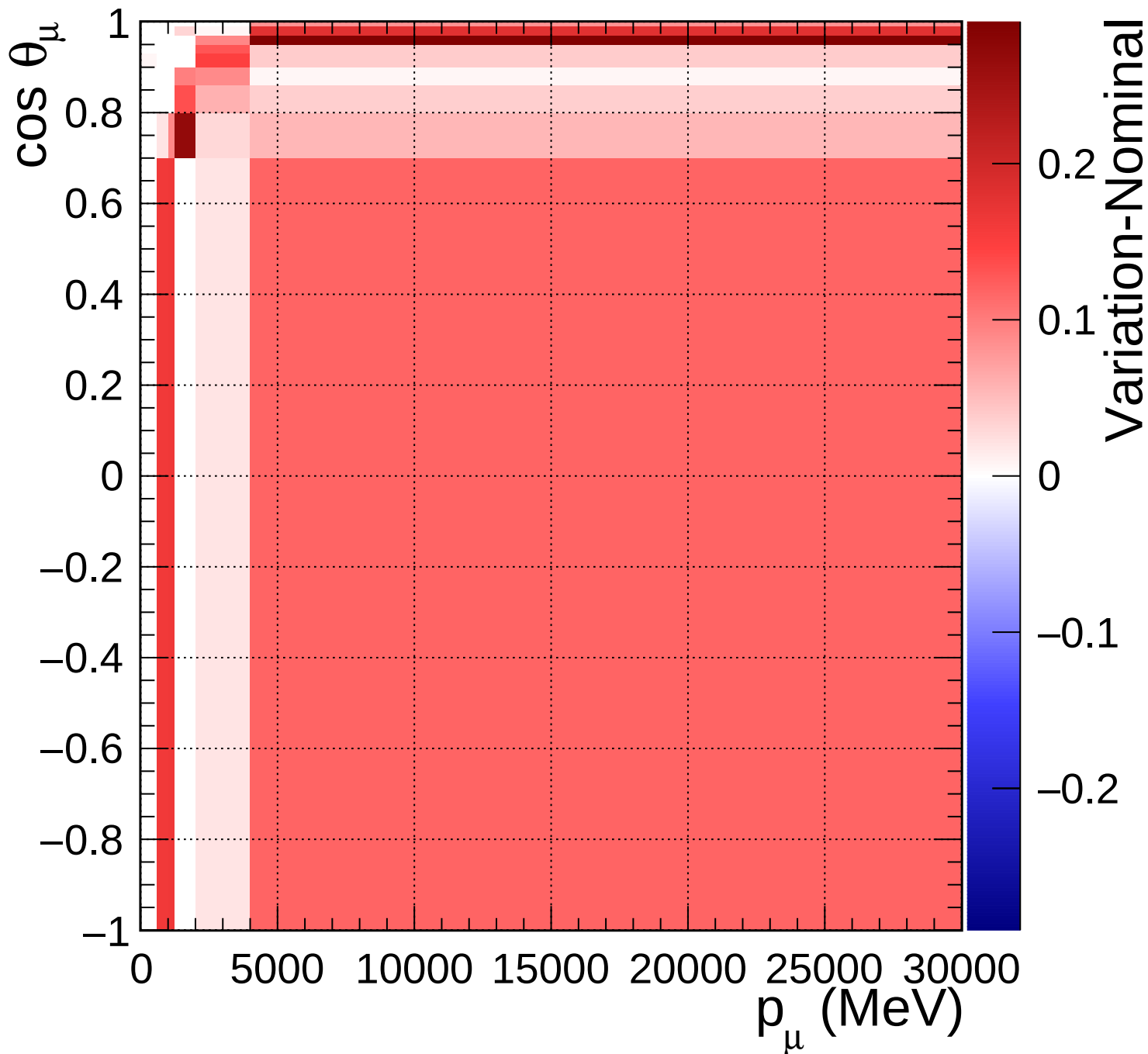
FGD1_NuMuBkg_CCoher_in_AntiNu_Mode_Q2_norm_7_1.4
