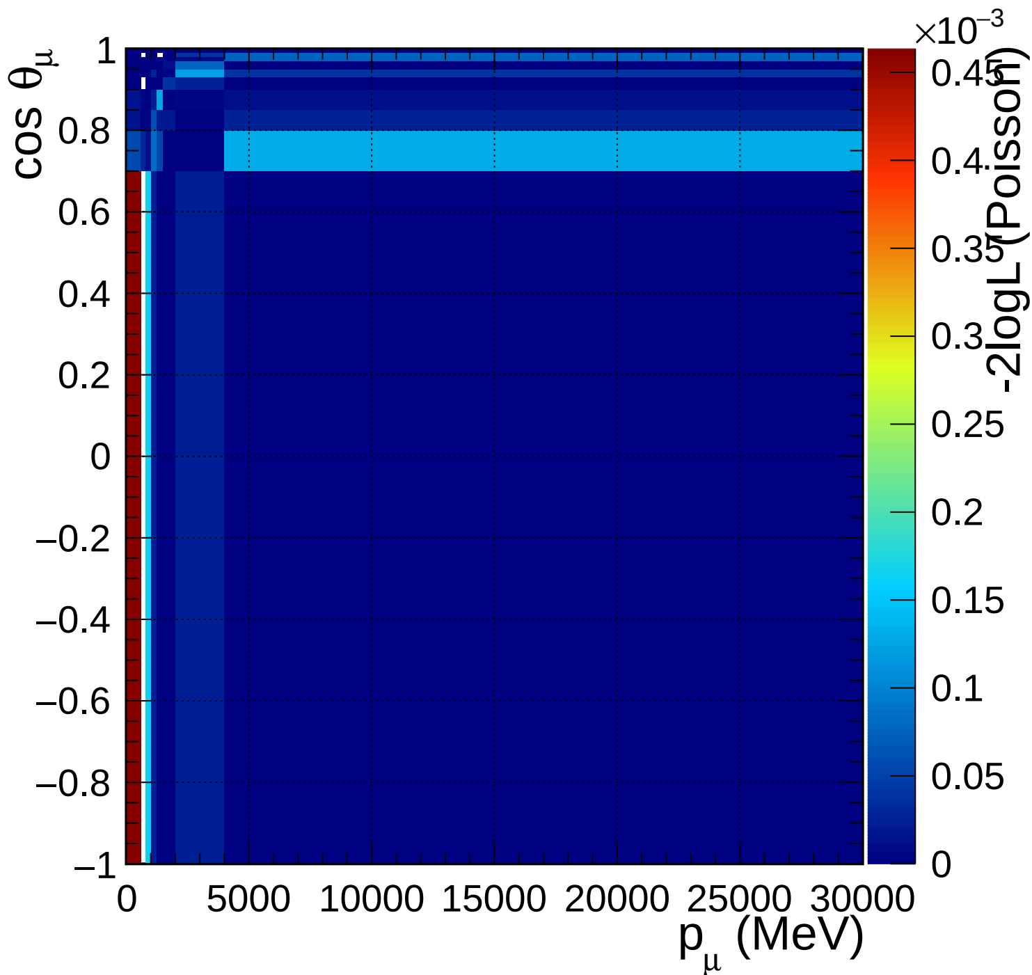
FGD1_anti-numuCC_other_Q2_norm_6_0.82
