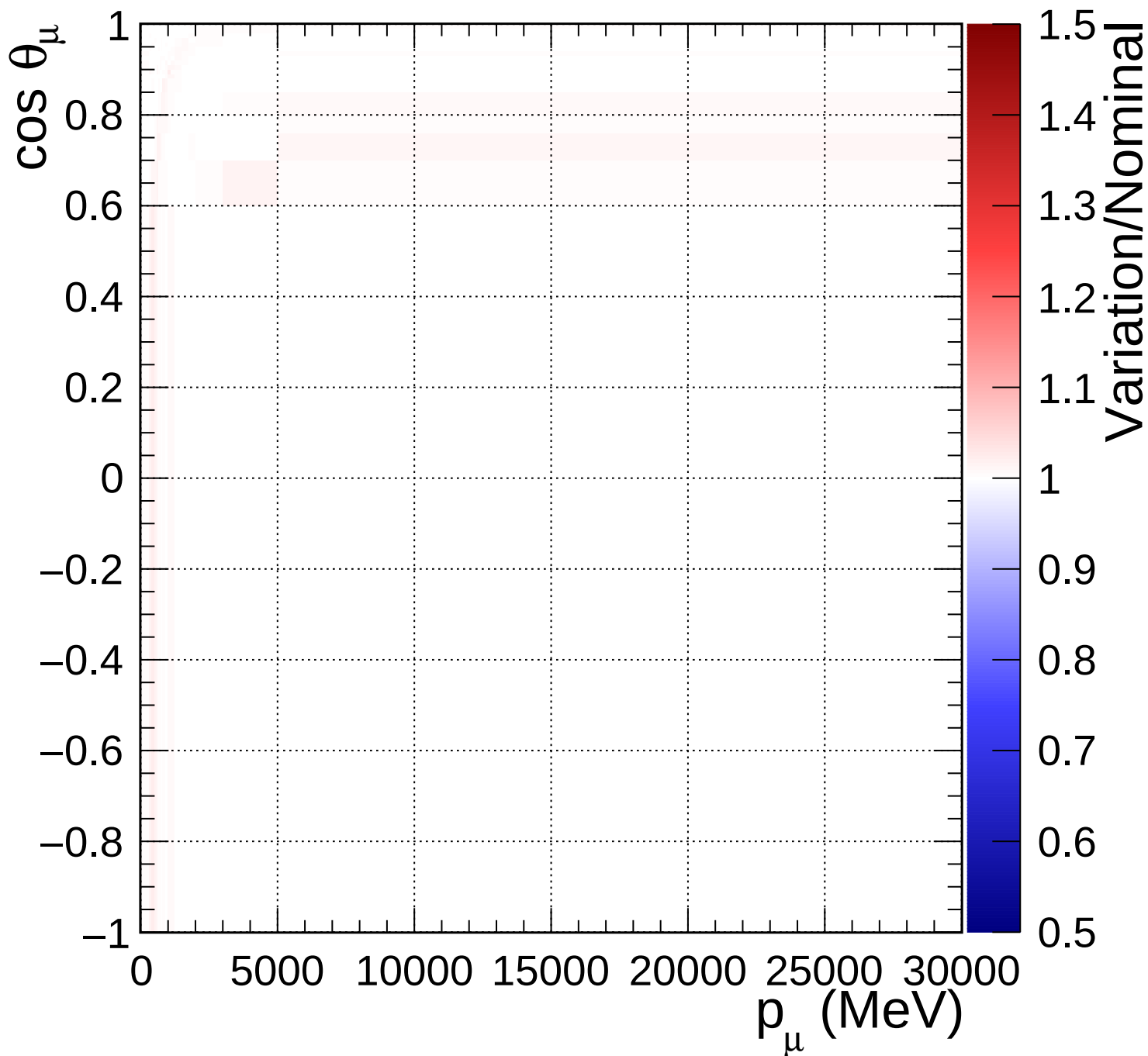
FGD2_numuCC_other_Q2_norm_5_1.33
