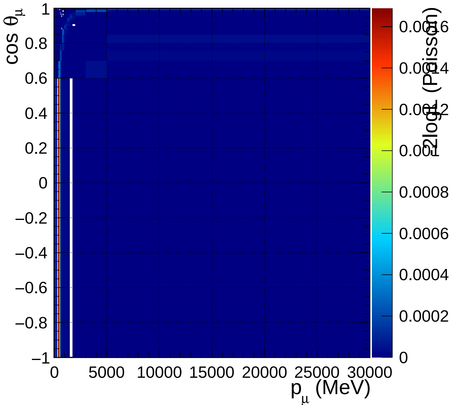
FGD2_numuCC_other_Q2_norm_5_1.11
