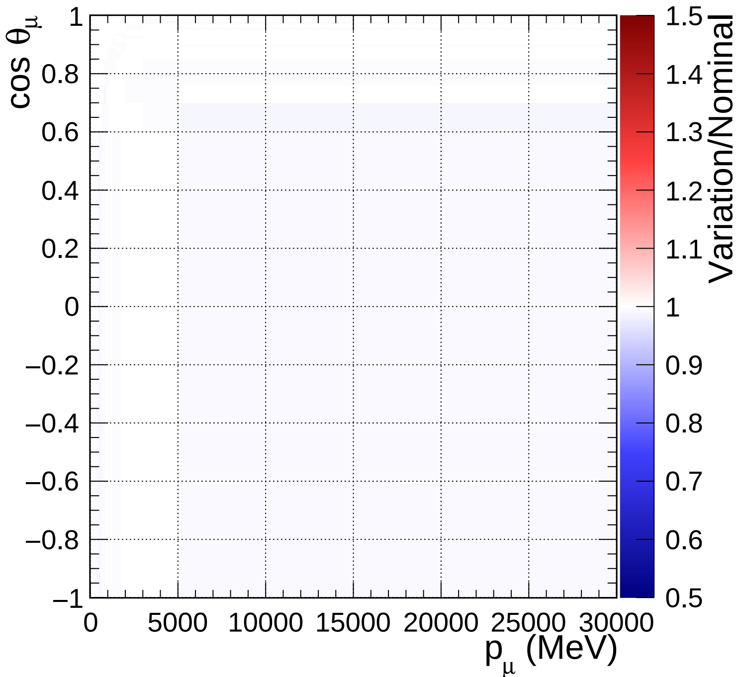
FGD2_numuCC_other_Q2_norm_6_0.82
