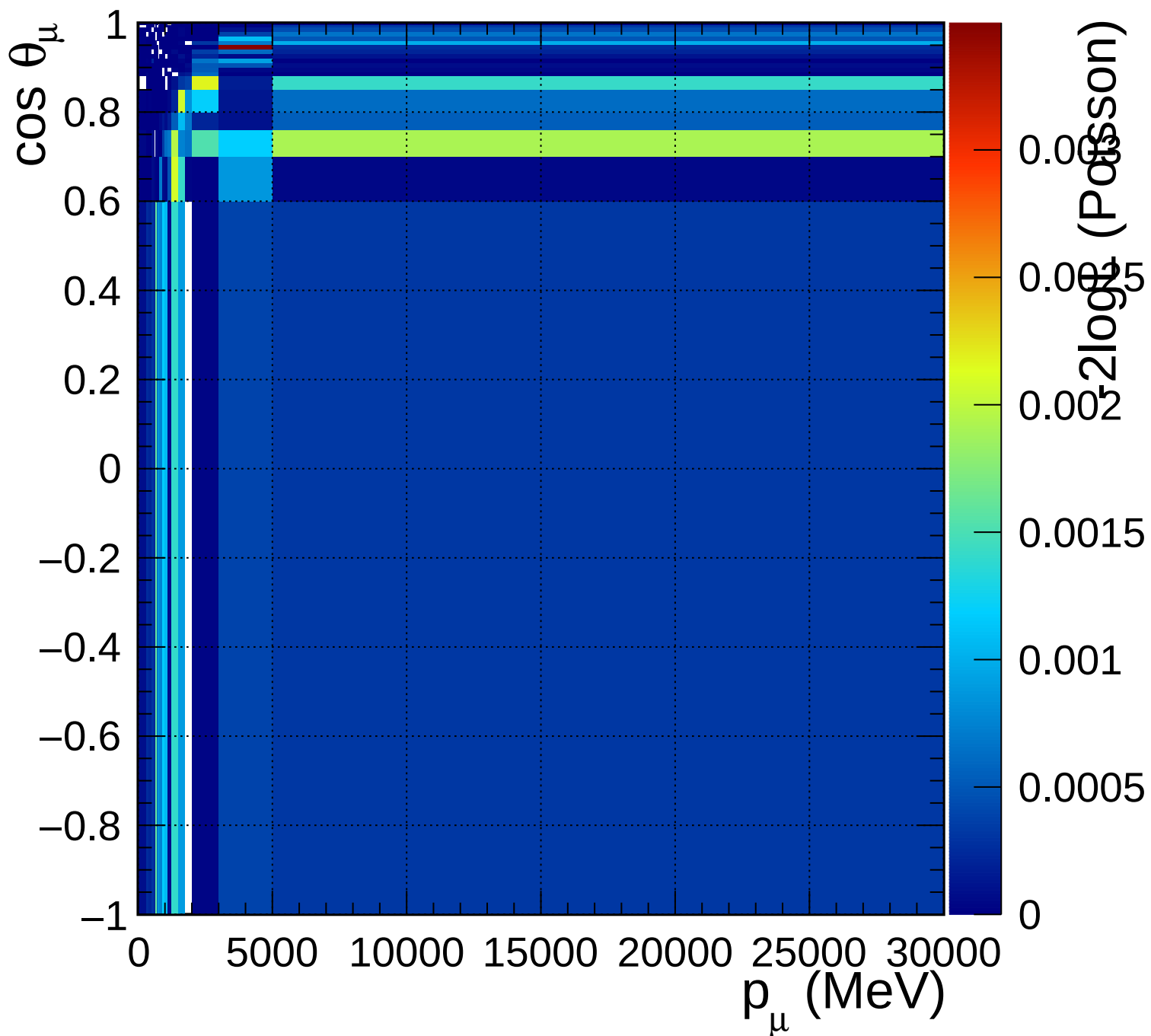
FGD2_numuCC_other_Q2_norm_7_1.4
