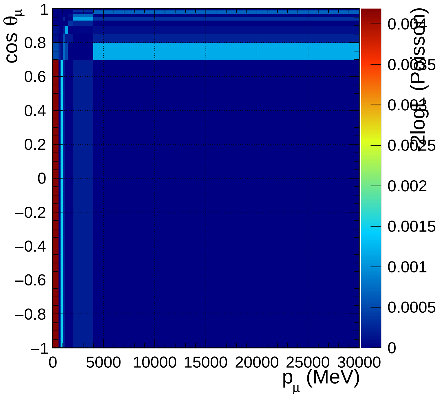
FGD1_anti-numuCC_other_Q2_norm_6_0.46
