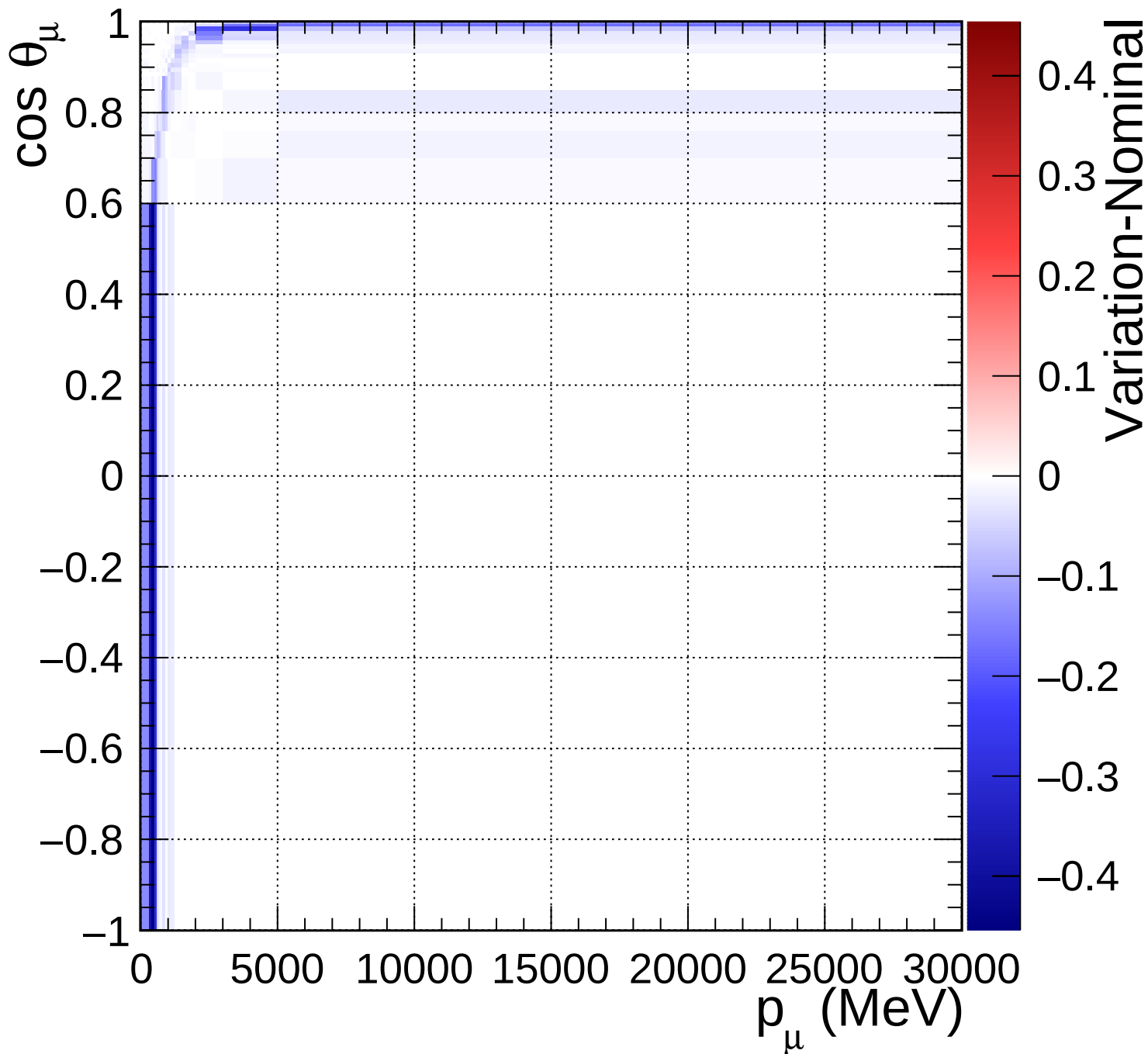
FGD2_numuCC_other_Q2_norm_5_0.89
