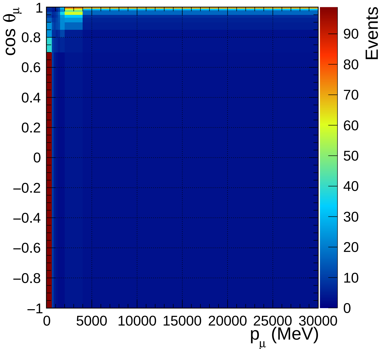
FGD1_anti-numuCC_other_Q2_norm_7_1
