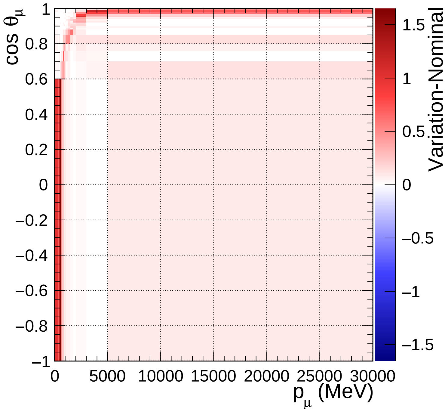
FGD2_numuCC_other_Q2_norm_6_1.54
