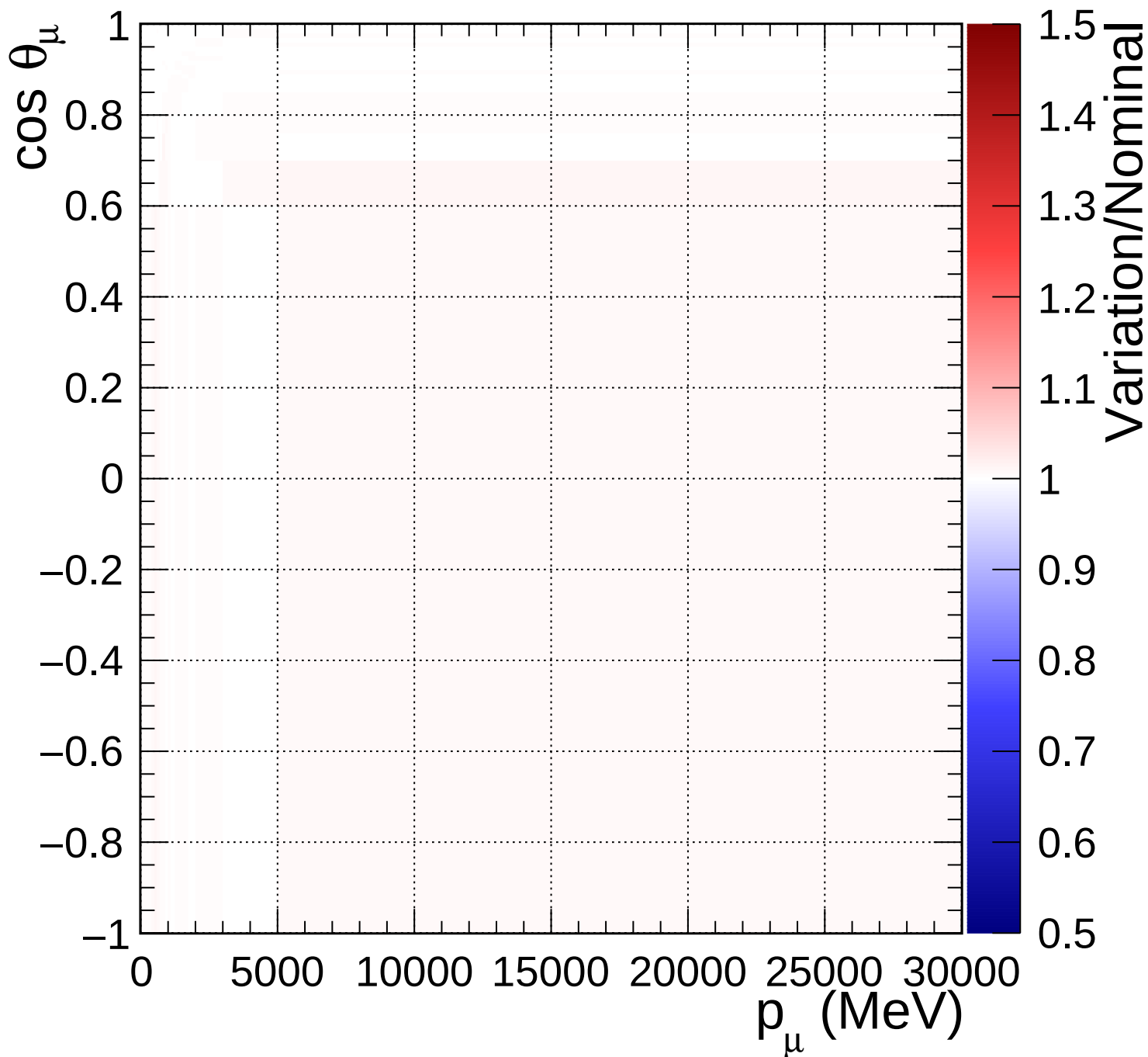
FGD2_numuCC_other_Q2_norm_6_1.18
