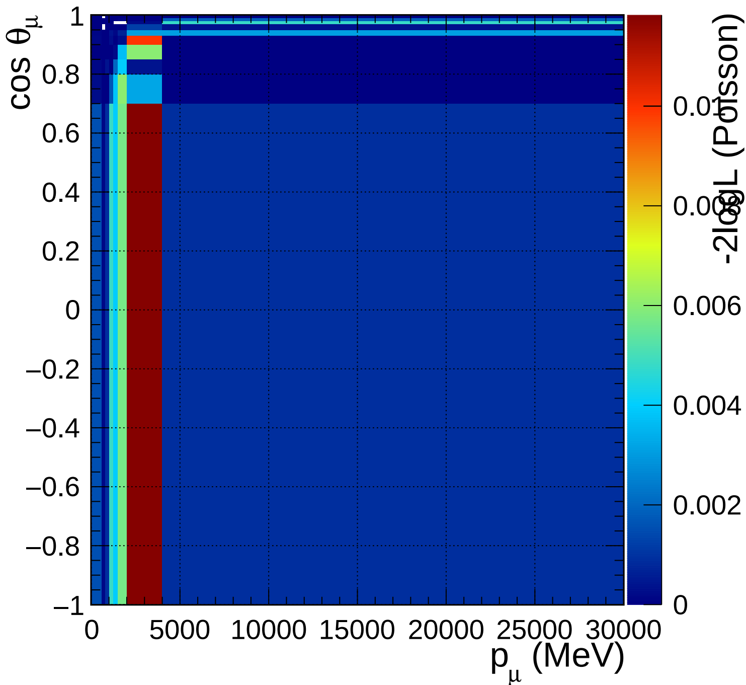
FGD1_anti-numuCC_other_Q2_norm_7_-0.2
