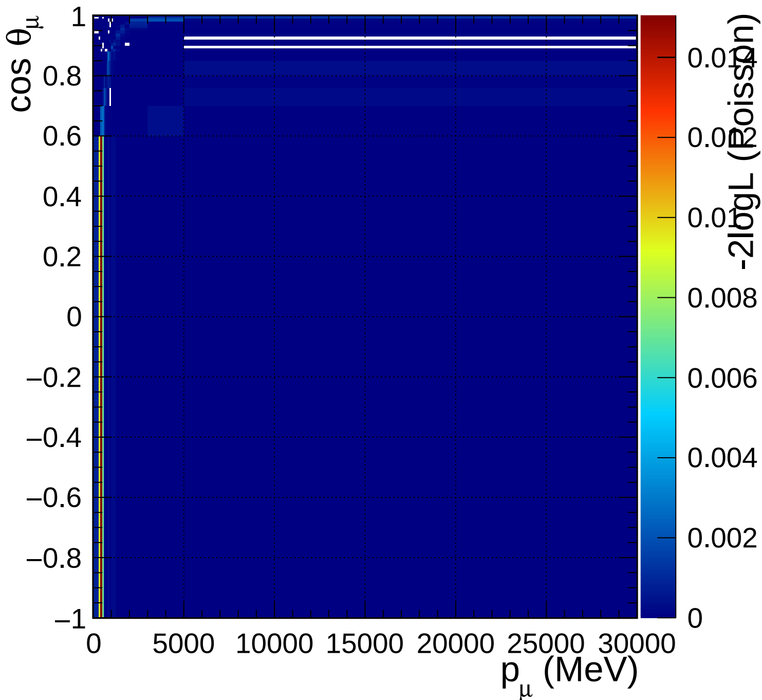
FGD2_numuCC_other_Q2_norm_5_1.33
