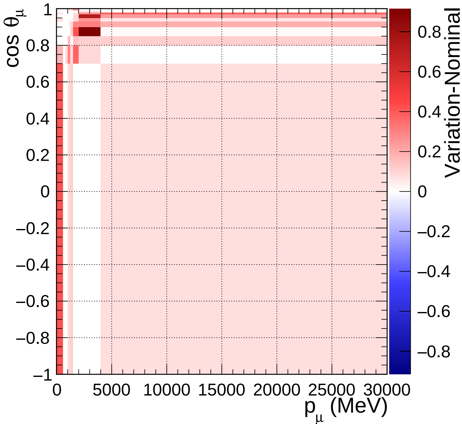
FGD2_anti-numuCC_other_Q2_norm_7_2.2
