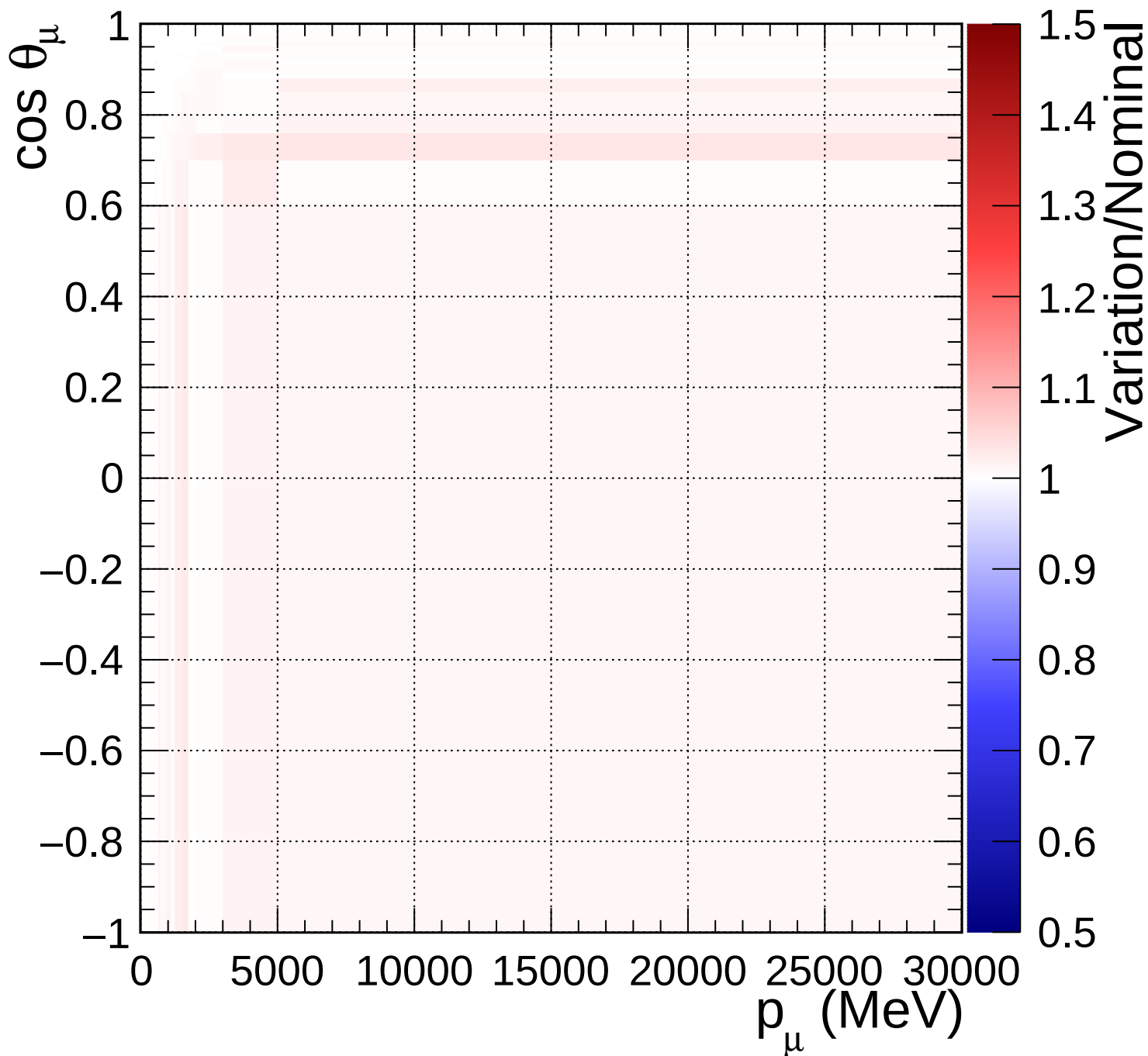
FGD2_numuCC_other_Q2_norm_7_1.4
