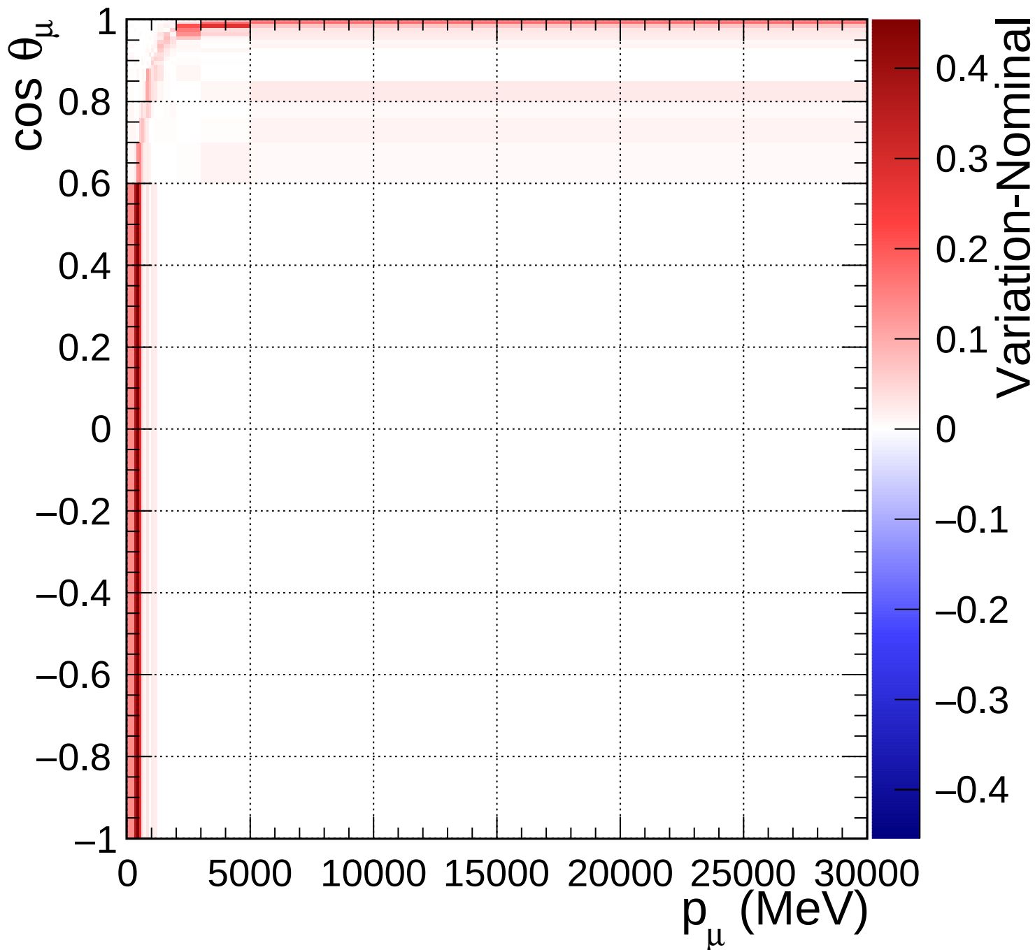
FGD2_numuCC_other_Q2_norm_5_1.11
