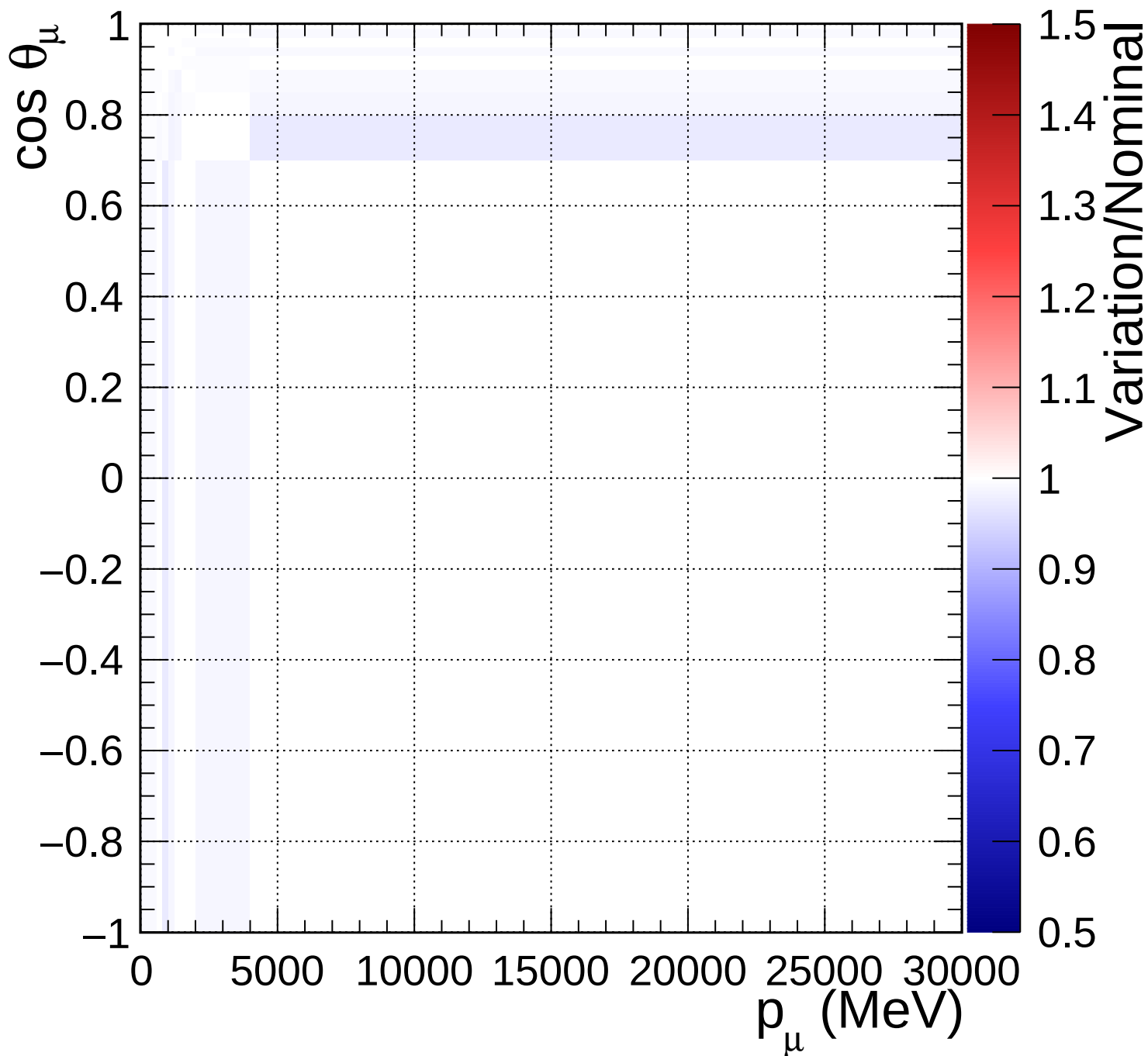
FGD1_anti-numuCC_other_Q2_norm_6_0.46
