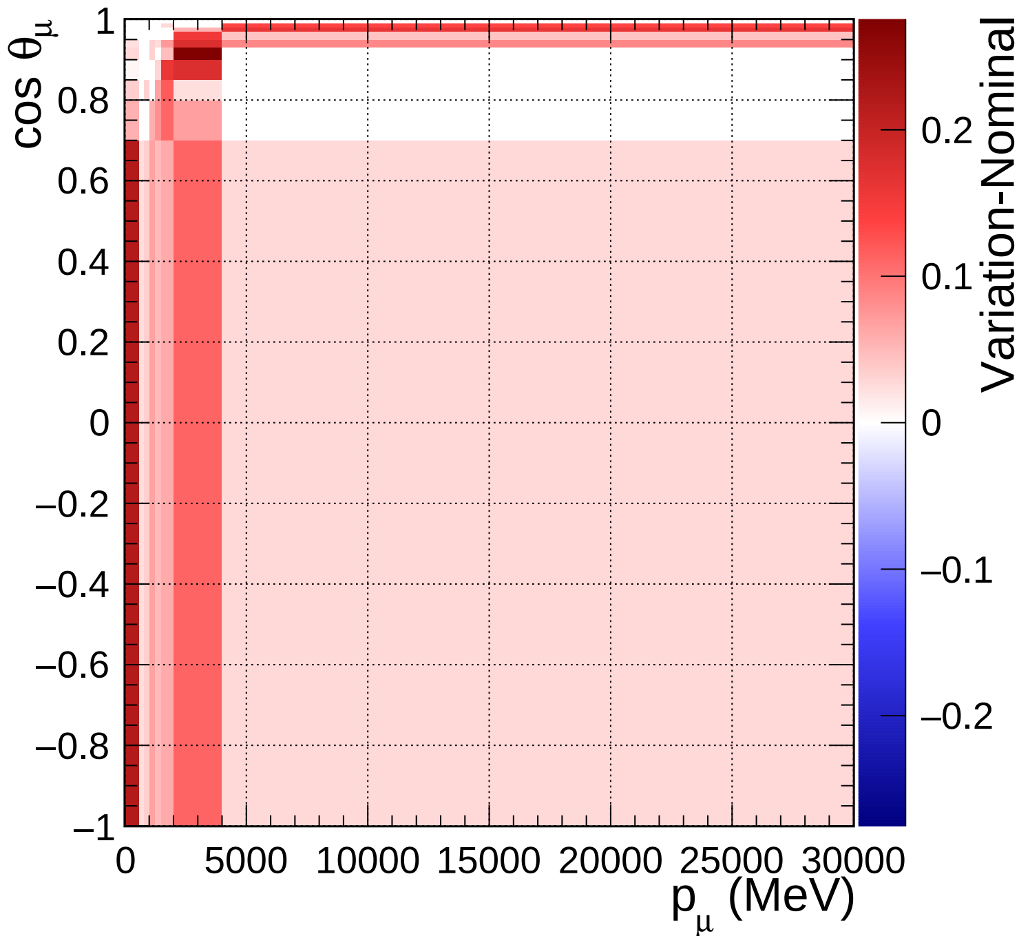
FGD1_anti-numuCC_other_Q2_norm_7_1.4
