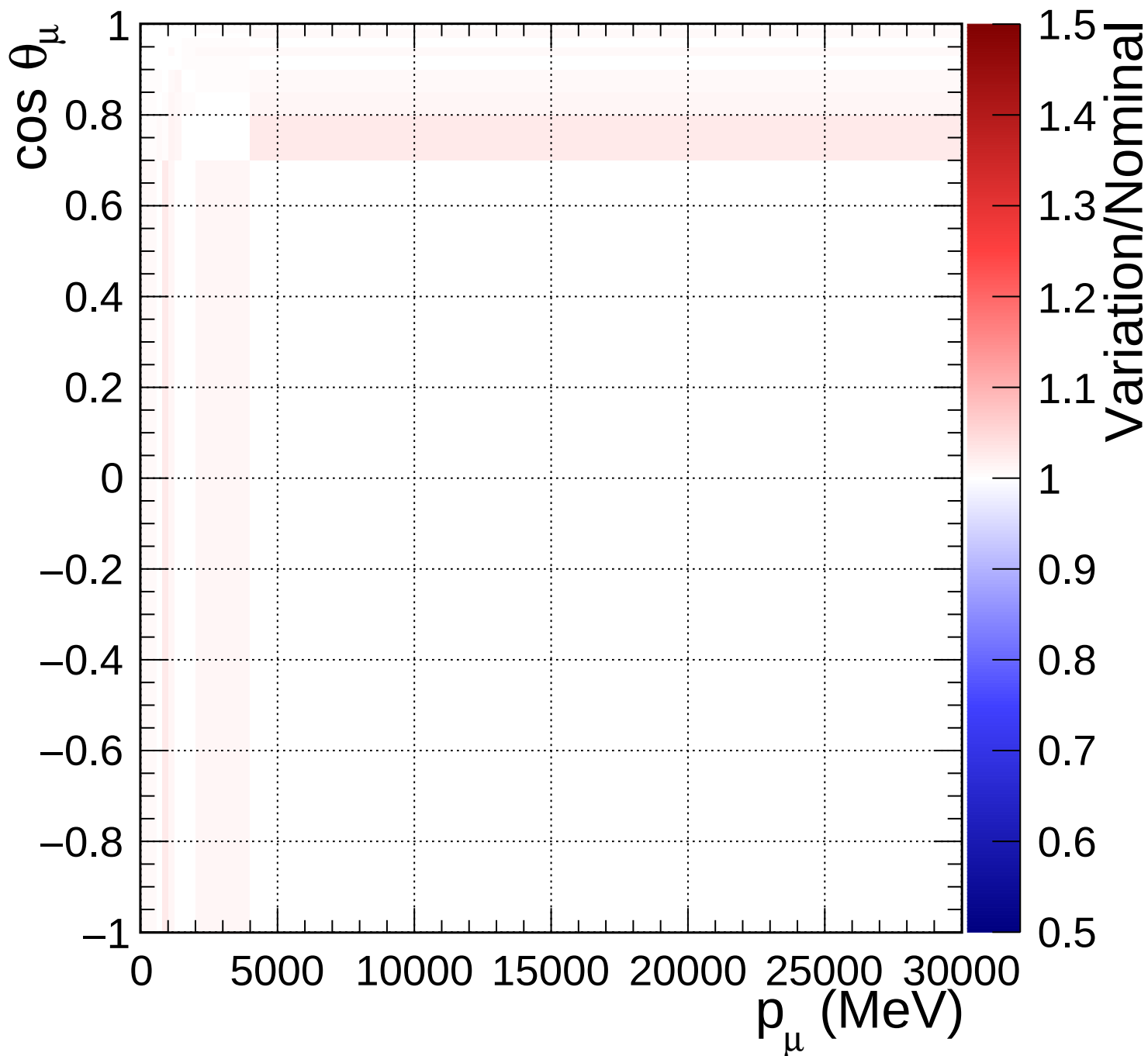
FGD1_anti-numuCC_other_Q2_norm_6_1.54
