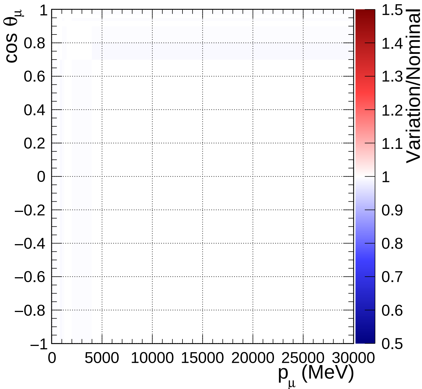
FGD1_anti-numuCC_other_Q2_norm_6_0.82
