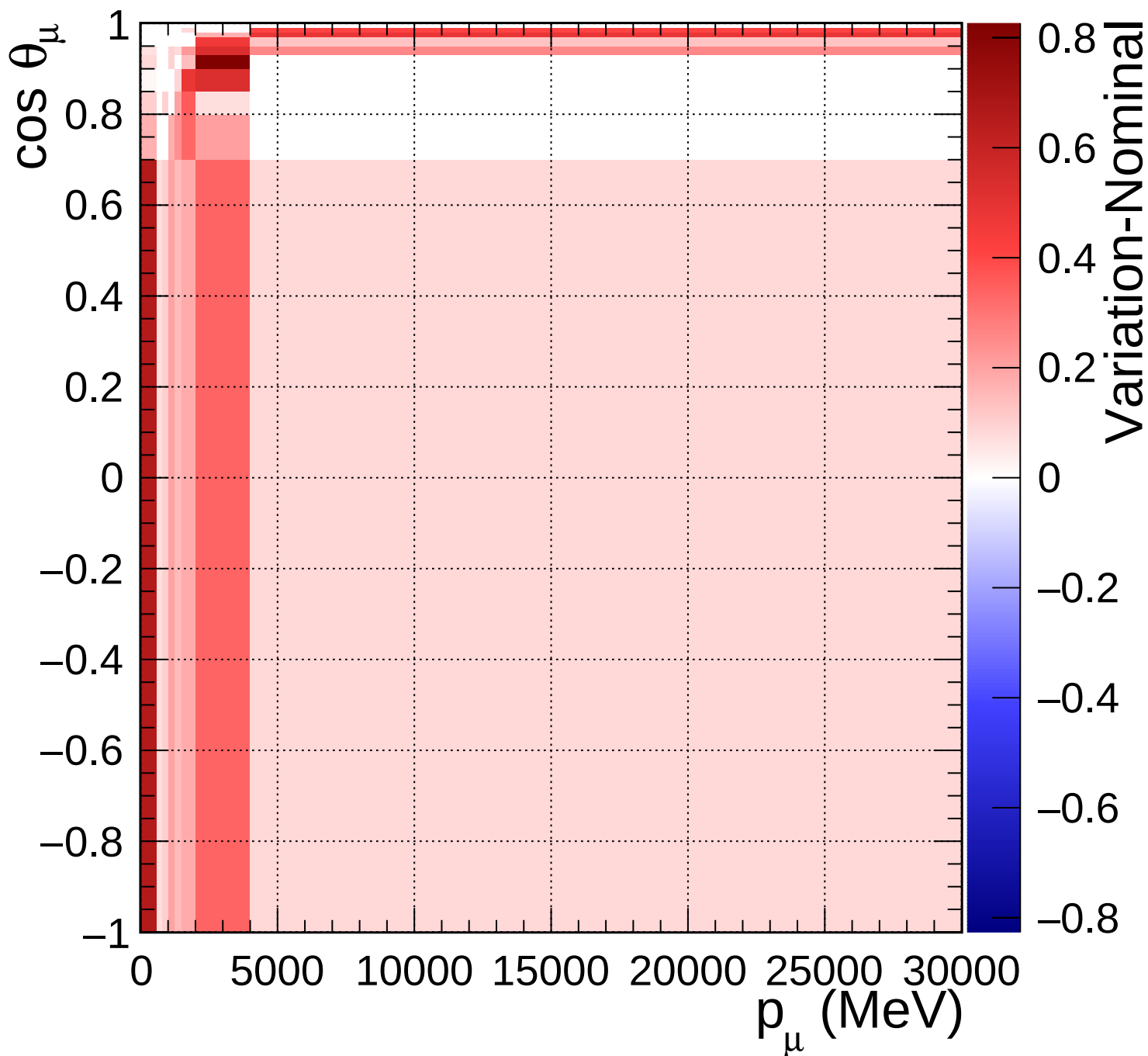
FGD1_anti-numuCC_other_Q2_norm_7_2.2
