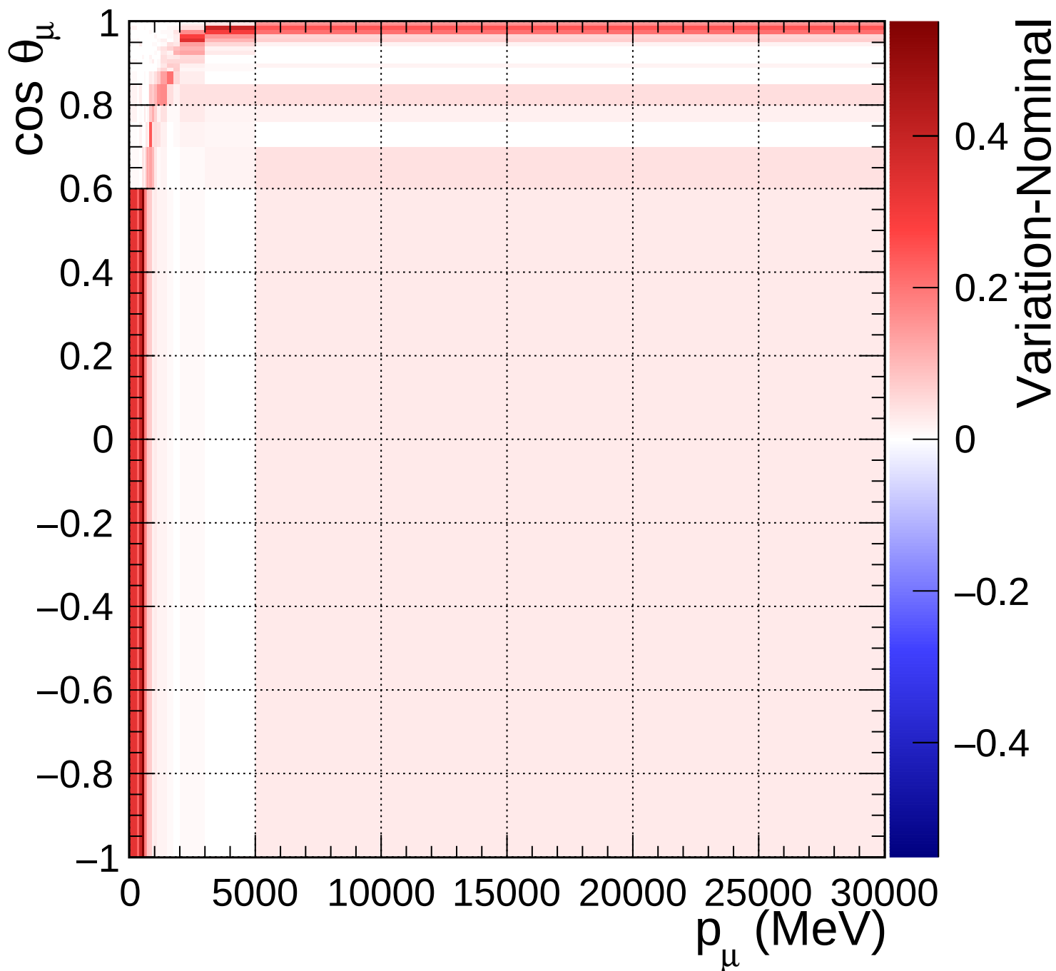
FGD2_numuCC_other_Q2_norm_6_1.18
