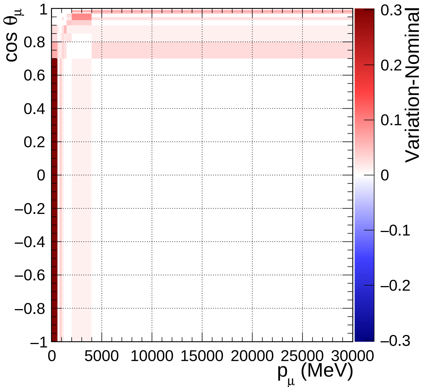
FGD1_anti-numuCC_other_Q2_norm_6_1.18
