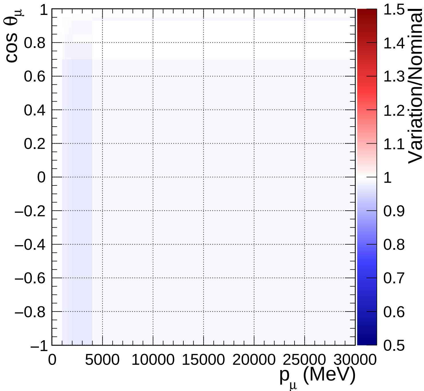
FGD1_anti-numuCC_other_Q2_norm_7_0.6
