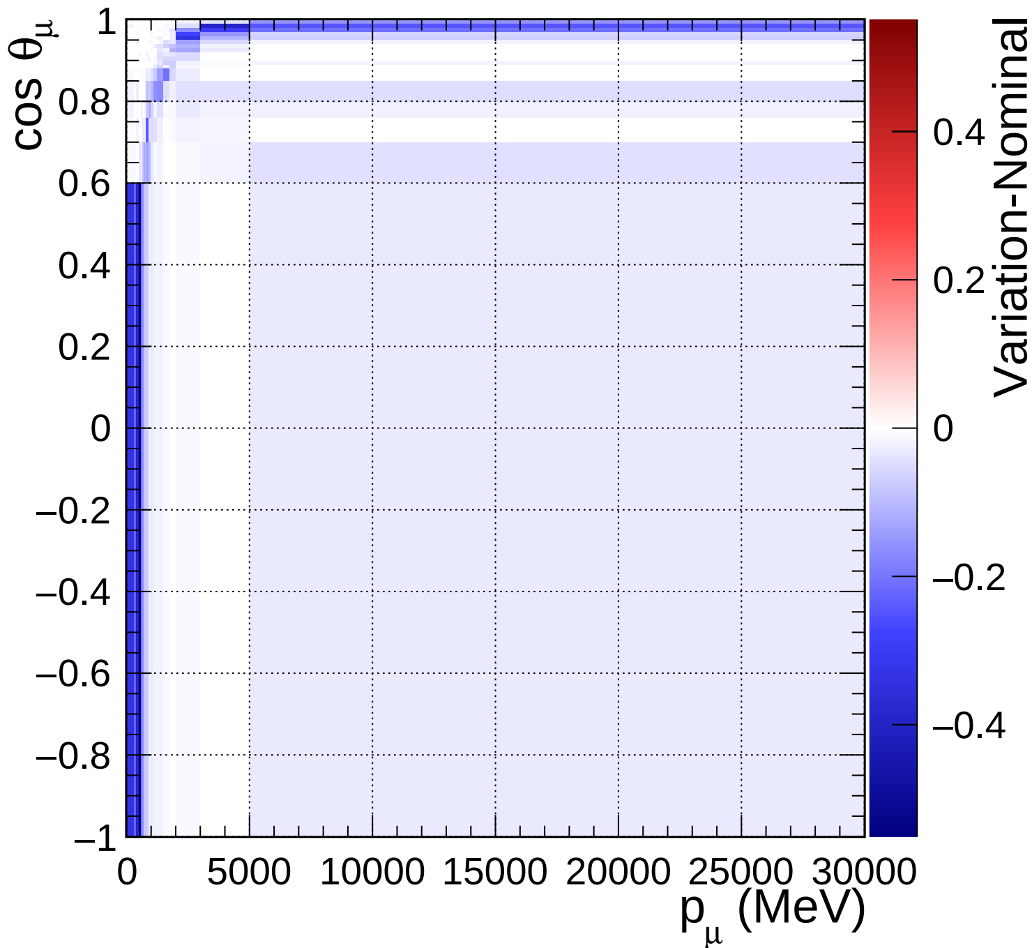
FGD2_numuCC_other_Q2_norm_6_0.82
