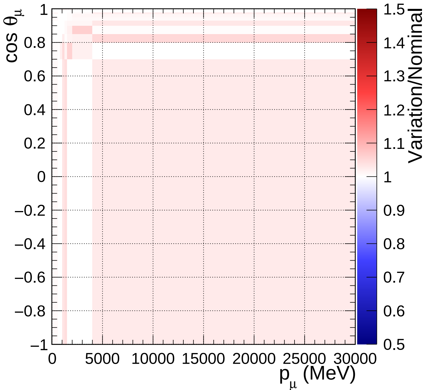
FGD2_anti-numuCC_other_Q2_norm_7_2.2
