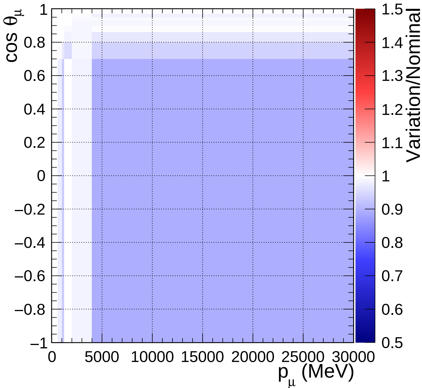
FGD1_NuMuBkg_CCoher_in_AntiNu_Mode_Q2_norm_7_-0.2
