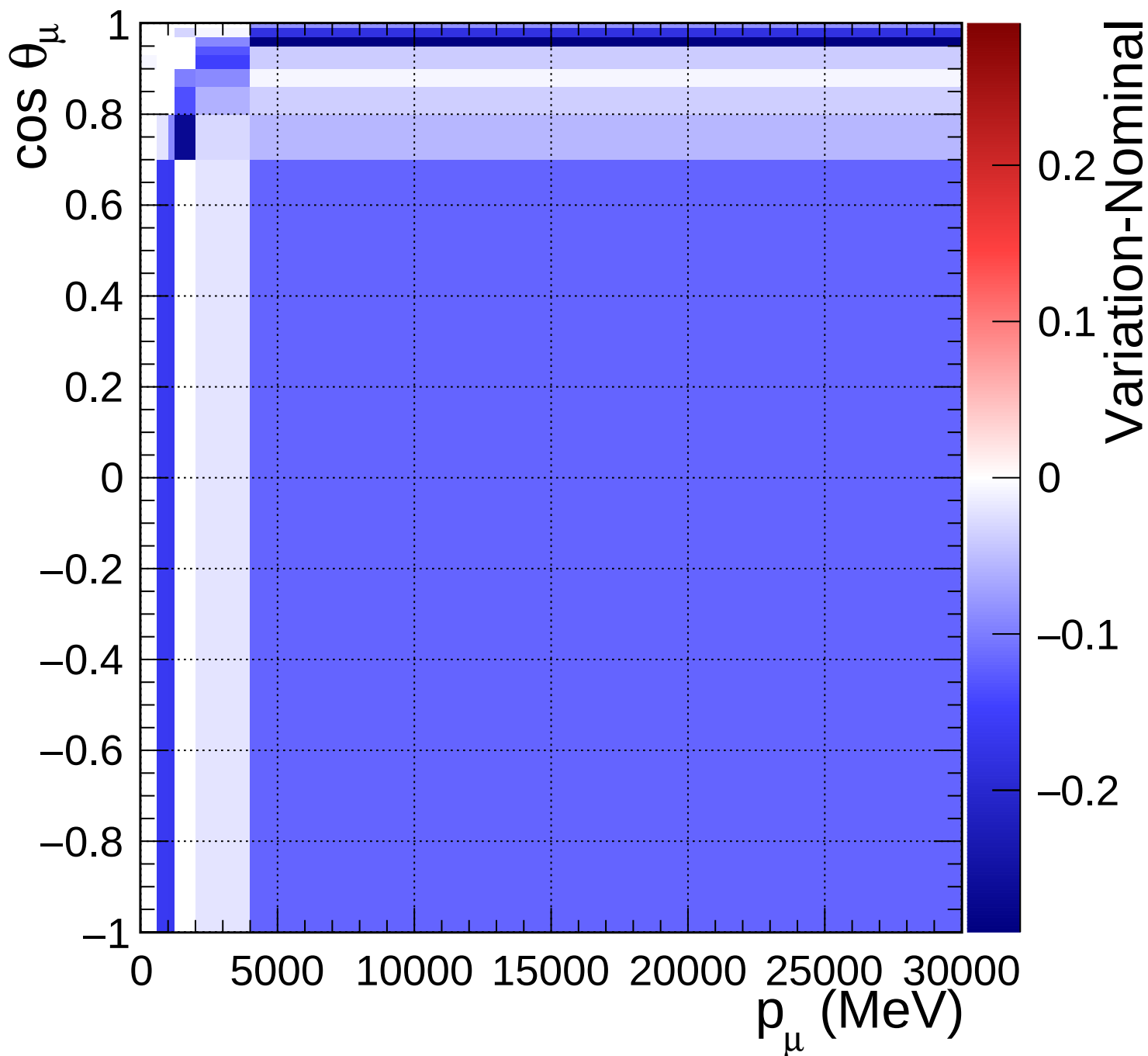
FGD1_NuMuBkg_CCoher_in_AntiNu_Mode_Q2_norm_7_0.6
