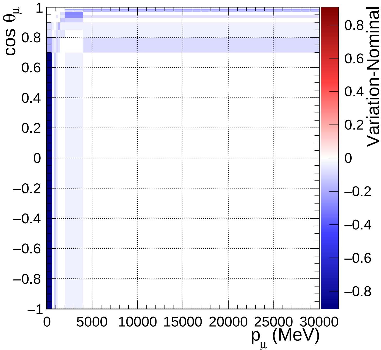
FGD1_anti-numuCC_other_Q2_norm_6_0.46
