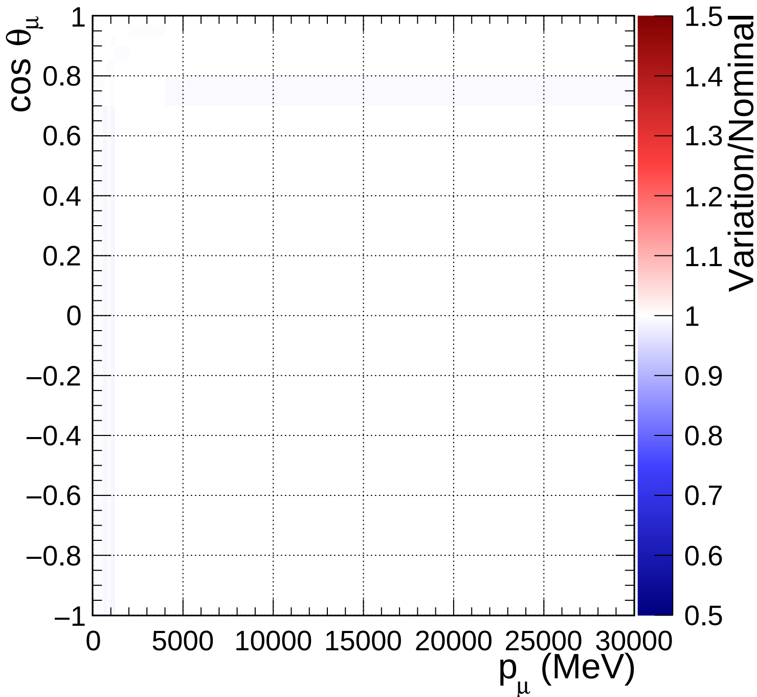
FGD2_anti-numuCC_other_Q2_norm_6_0.82
