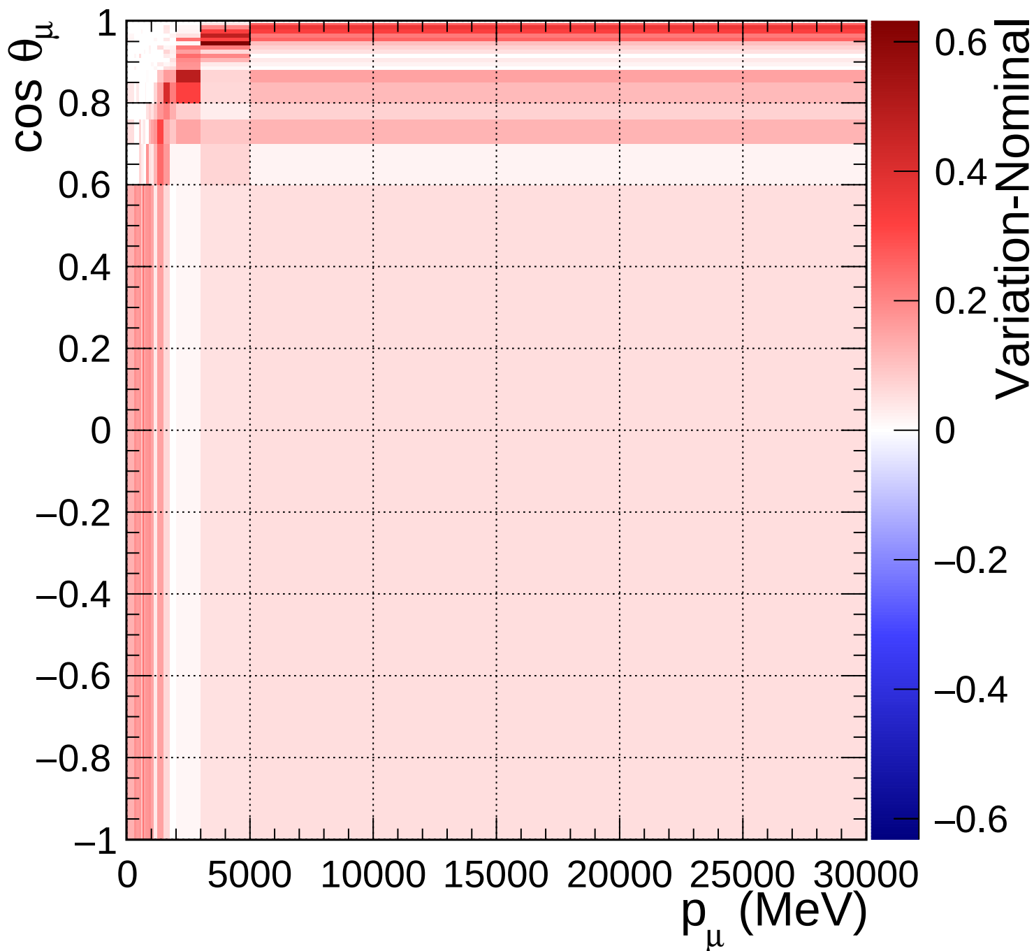
FGD2_numuCC_other_Q2_norm_7_1.4
