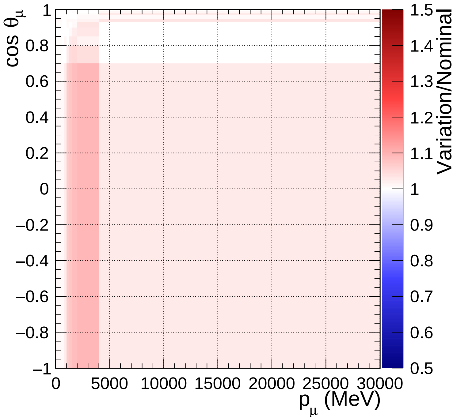
FGD1_anti-numuCC_other_Q2_norm_7_2.2
