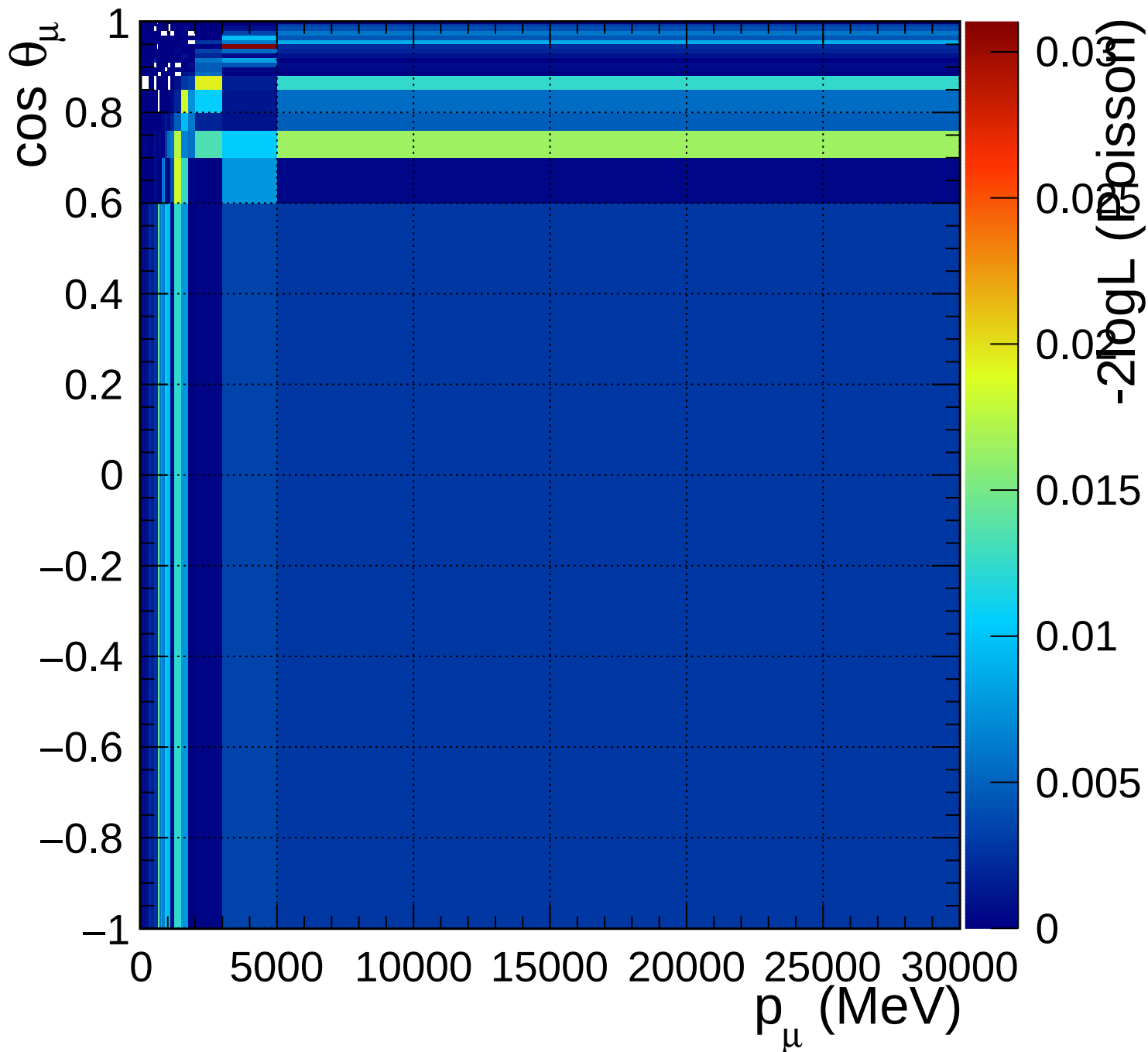
FGD2_numuCC_other_Q2_norm_7_2.2
