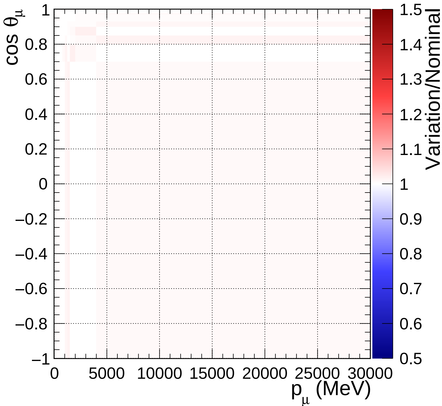
FGD2_anti-numuCC_other_Q2_norm_7_1.4
