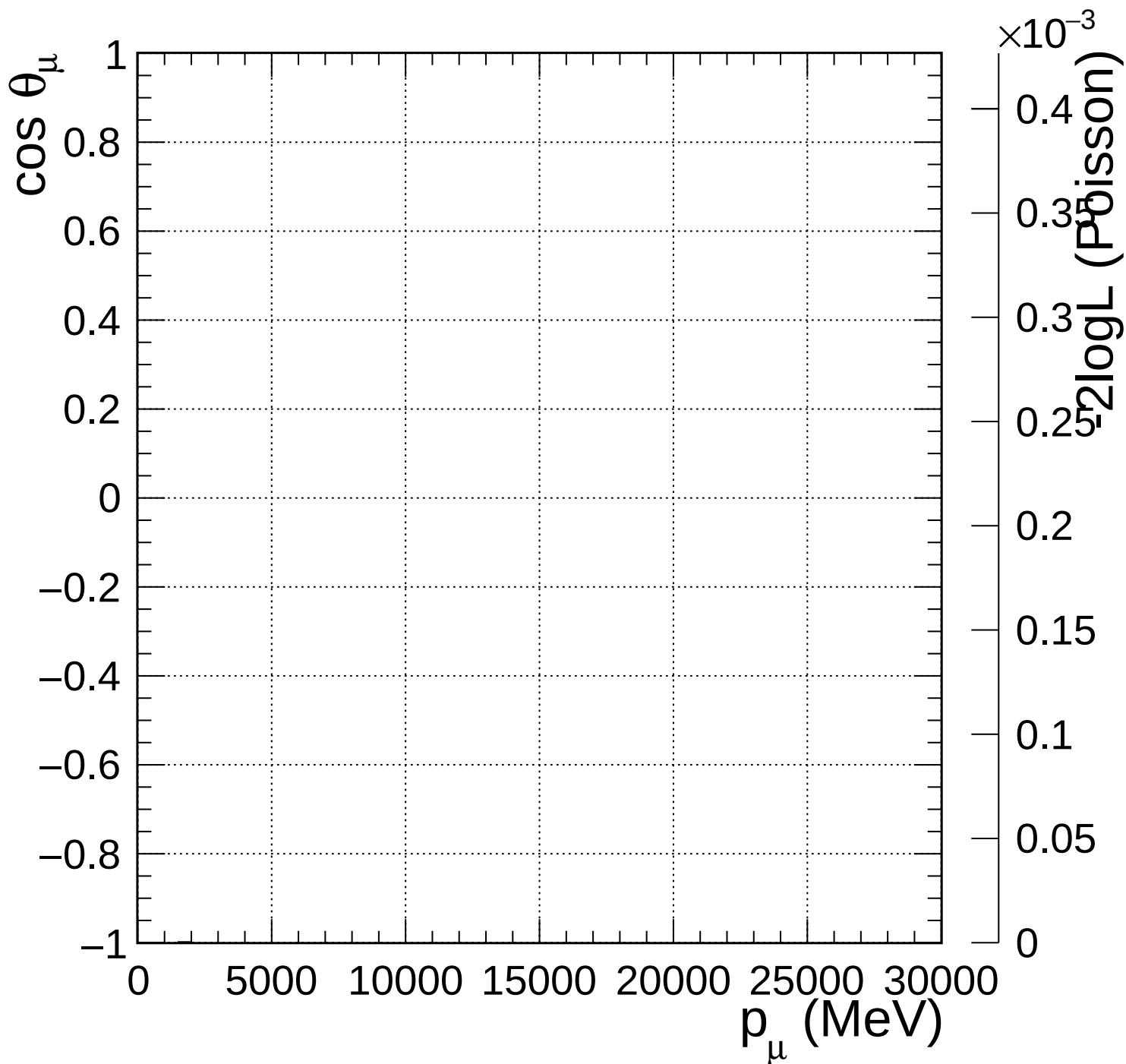
FGD2_anti-numuCC_other_Q2_norm_6_1.18
