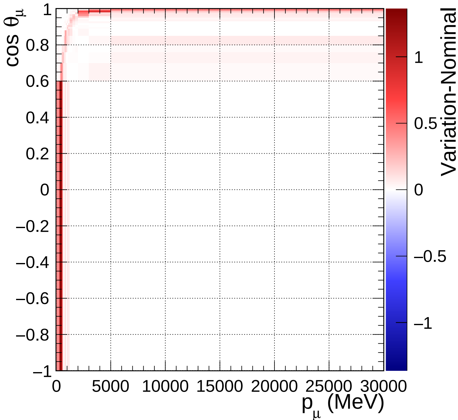
FGD2_numuCC_other_Q2_norm_5_1.33
