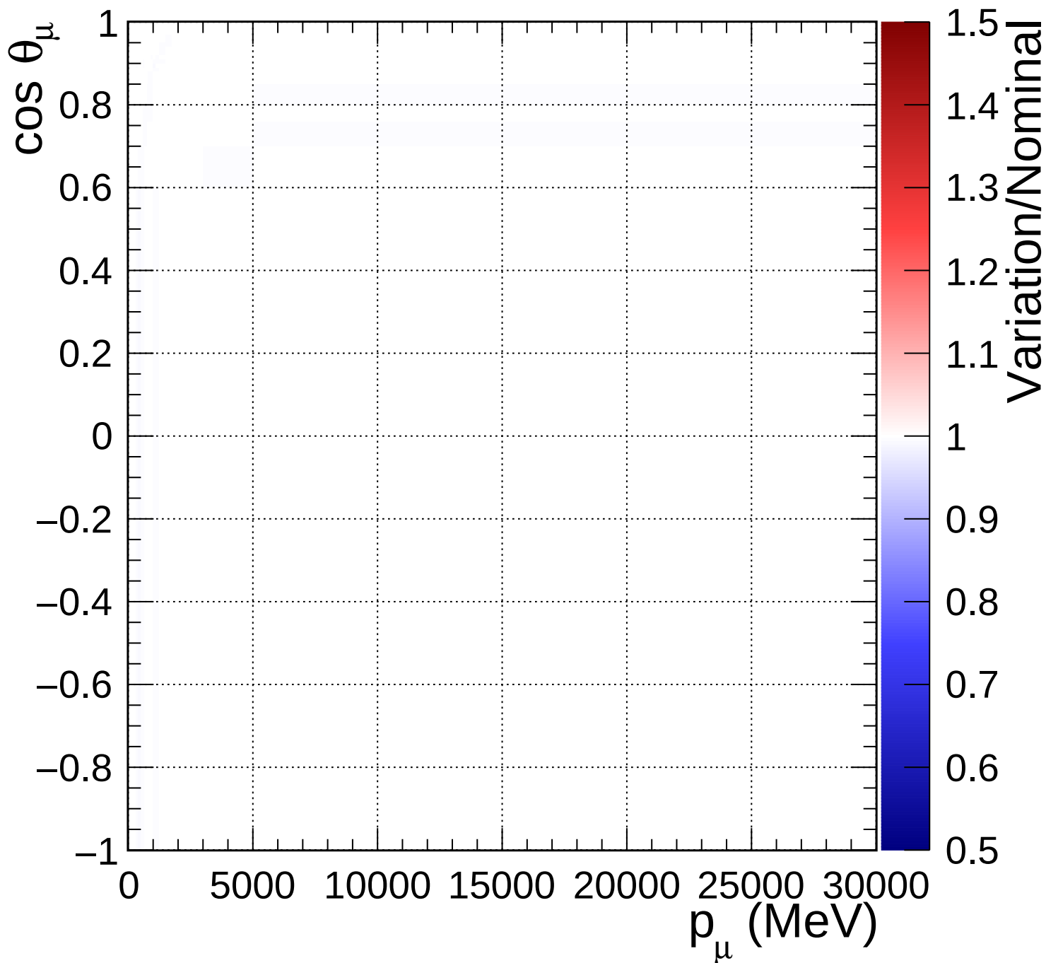
FGD2_numuCC_other_Q2_norm_5_0.89
