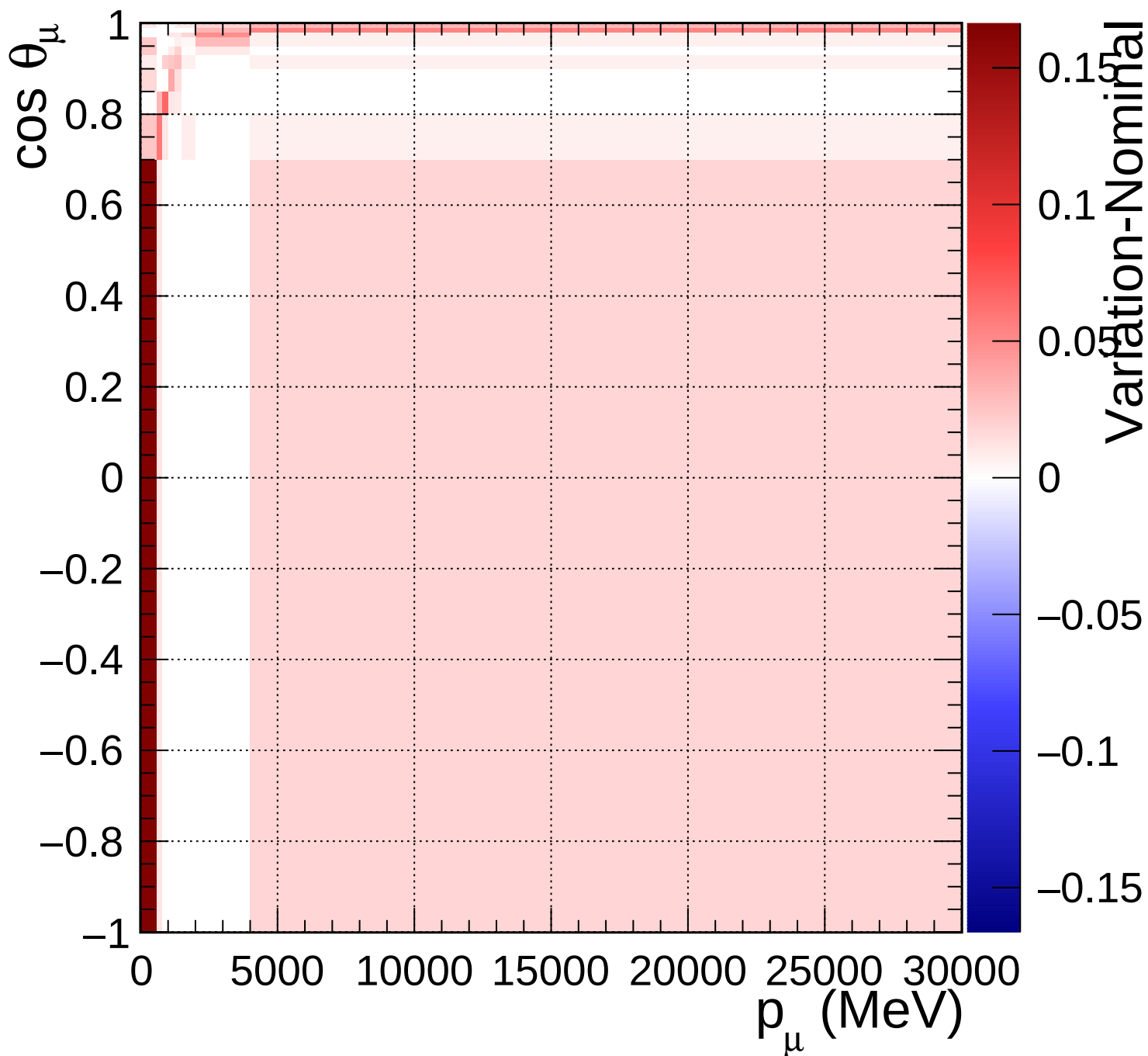
FGD2_anti-numuCC_other_Q2_norm_5_1.11
