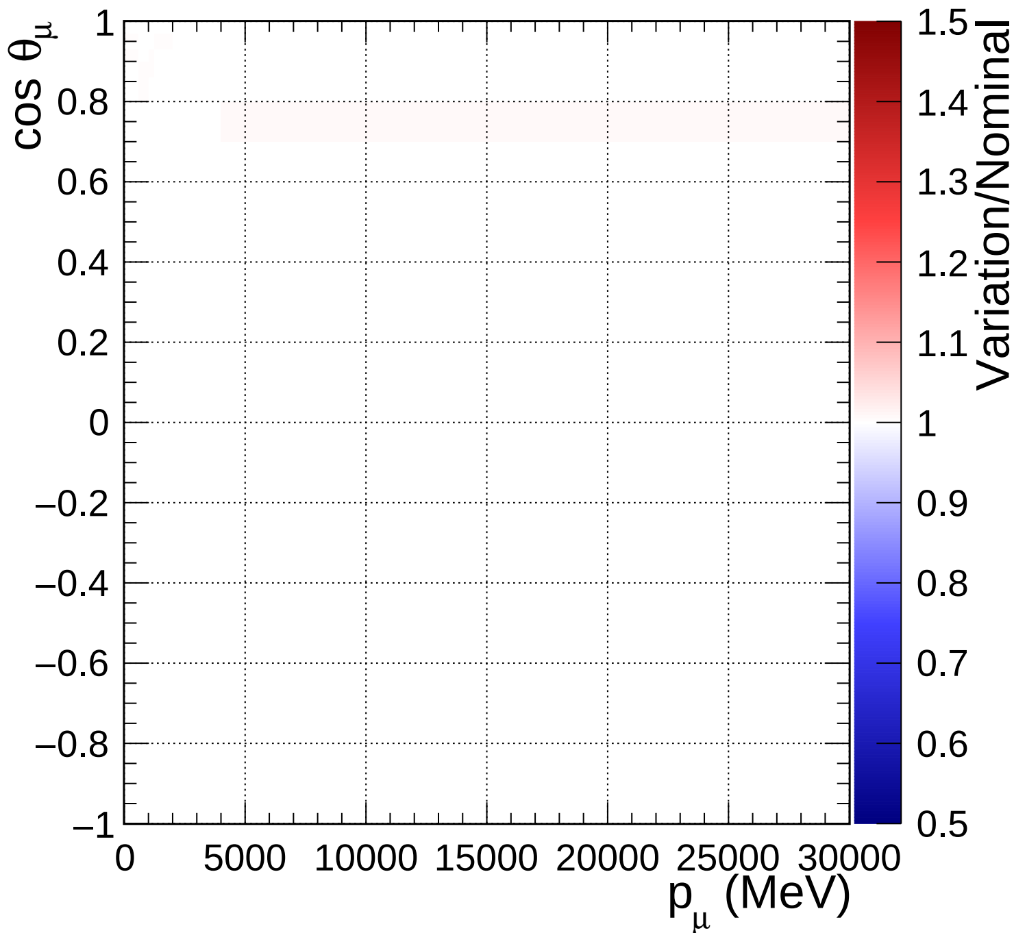
FGD1_NuMuBkg_CCoher_in_AntiNu_Mode_Q2_norm_5_1.11
