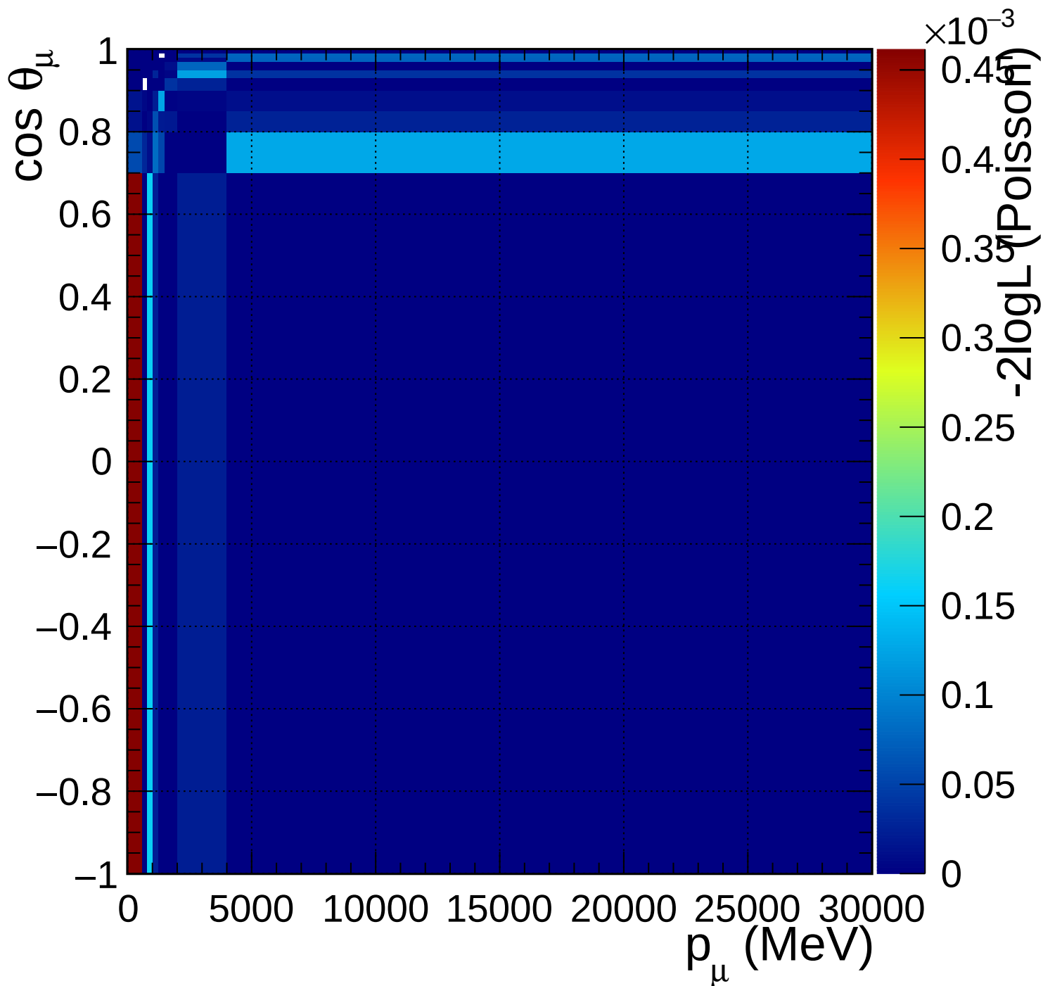
FGD1_anti-numuCC_other_Q2_norm_6_1.18
