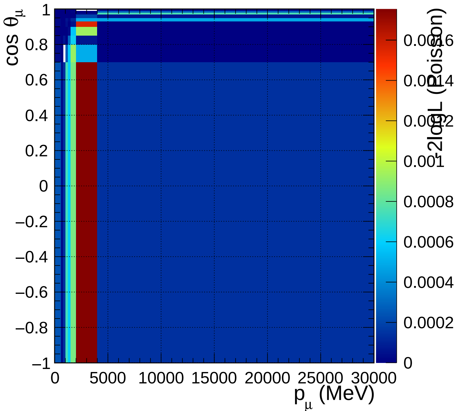
FGD1_anti-numuCC_other_Q2_norm_7_1.4
