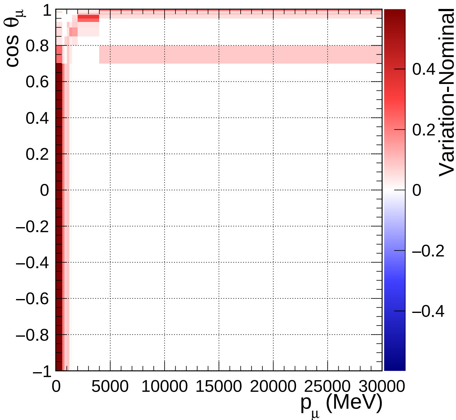
FGD2_anti-numuCC_other_Q2_norm_6_1.54
