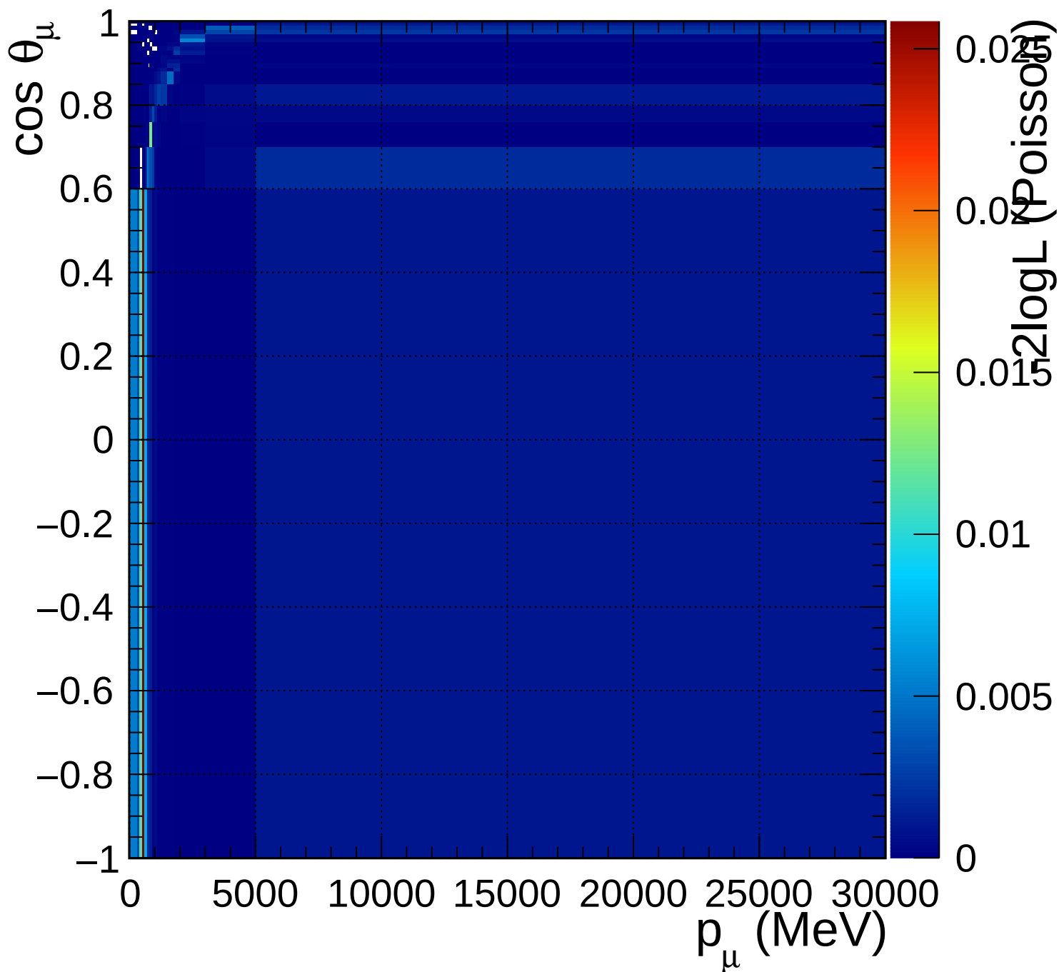
FGD2_numuCC_other_Q2_norm_6_1.54
