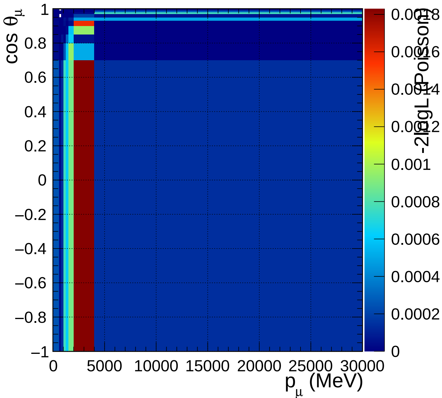
FGD1_anti-numuCC_other_Q2_norm_7_0.6
