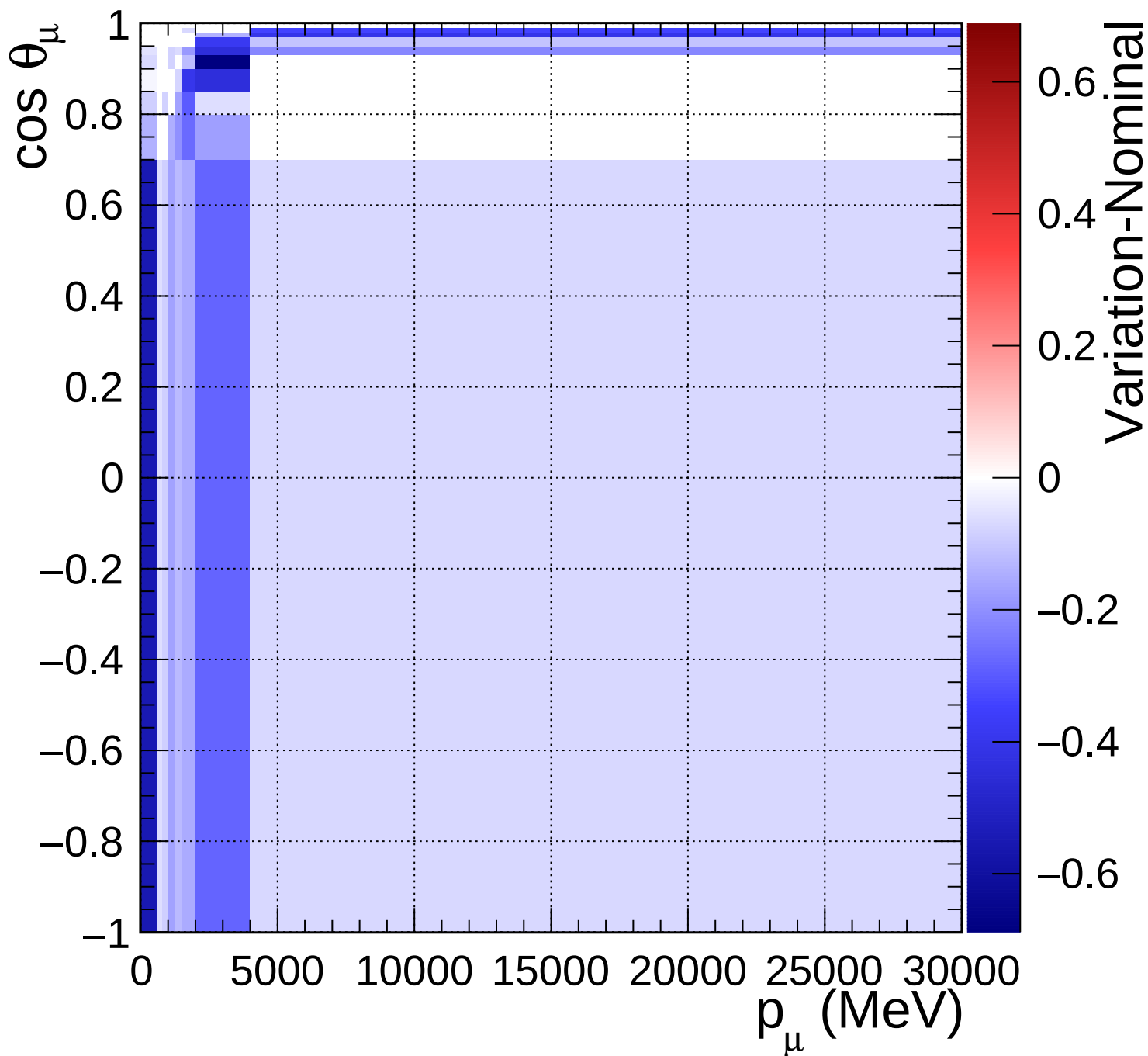
FGD1_anti-numuCC_other_Q2_norm_7_-0.2
