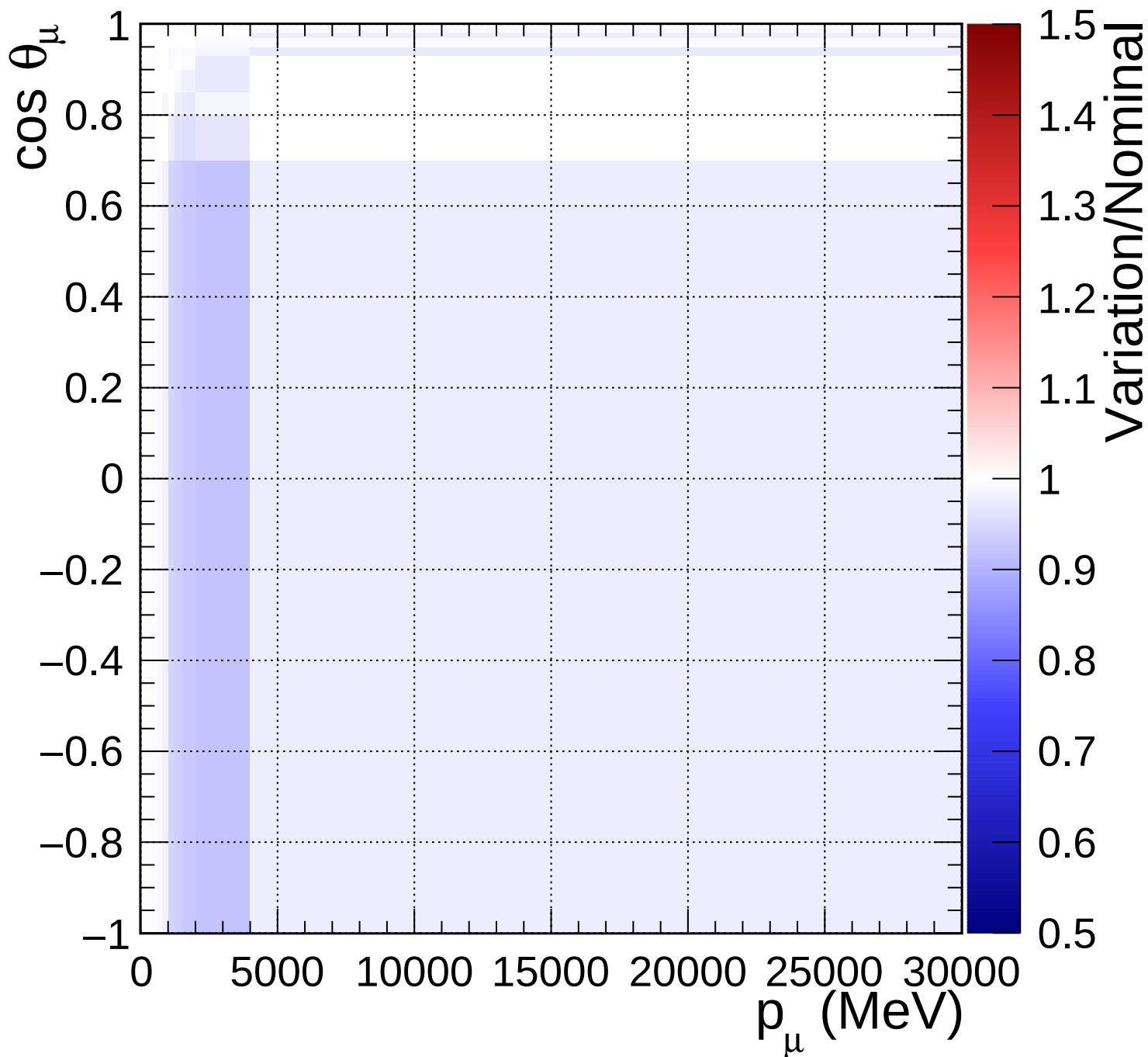
FGD1_anti-numuCC_other_Q2_norm_7_-0.2
