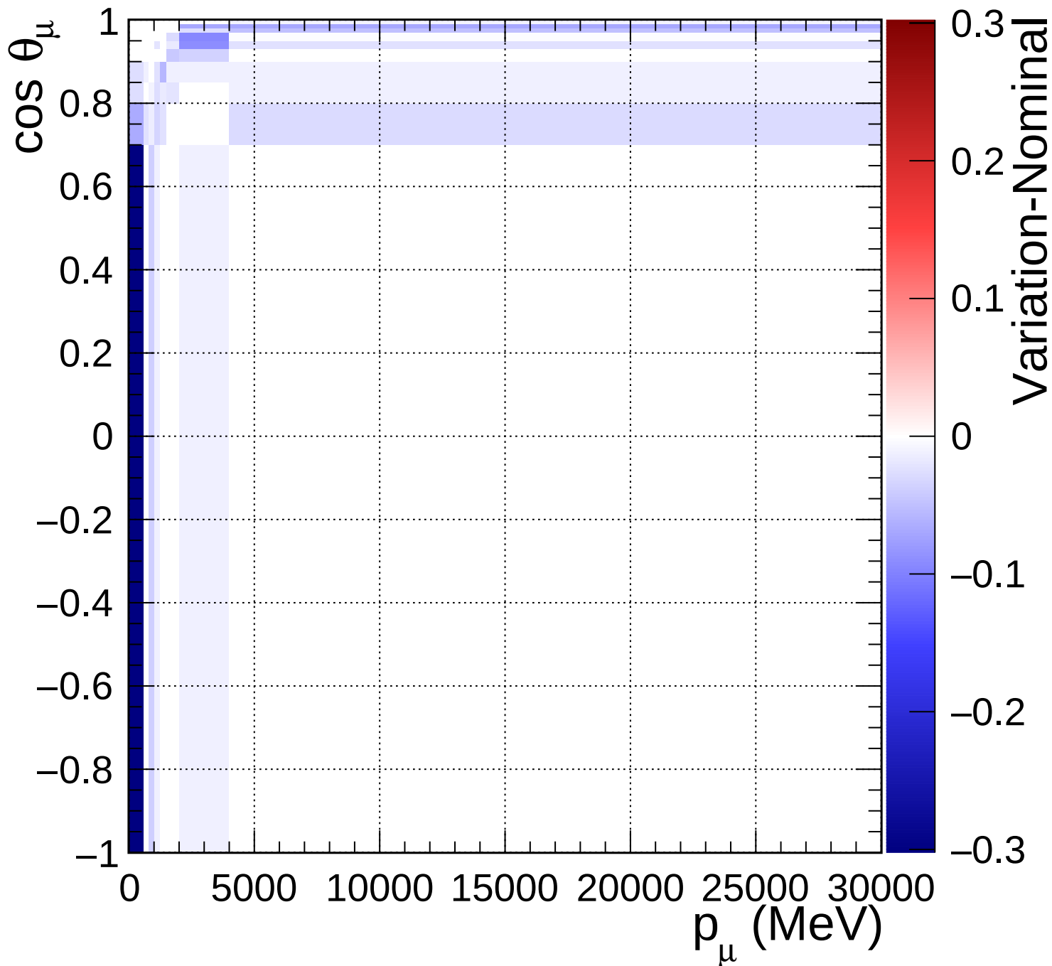
FGD1_anti-numuCC_other_Q2_norm_6_0.82
