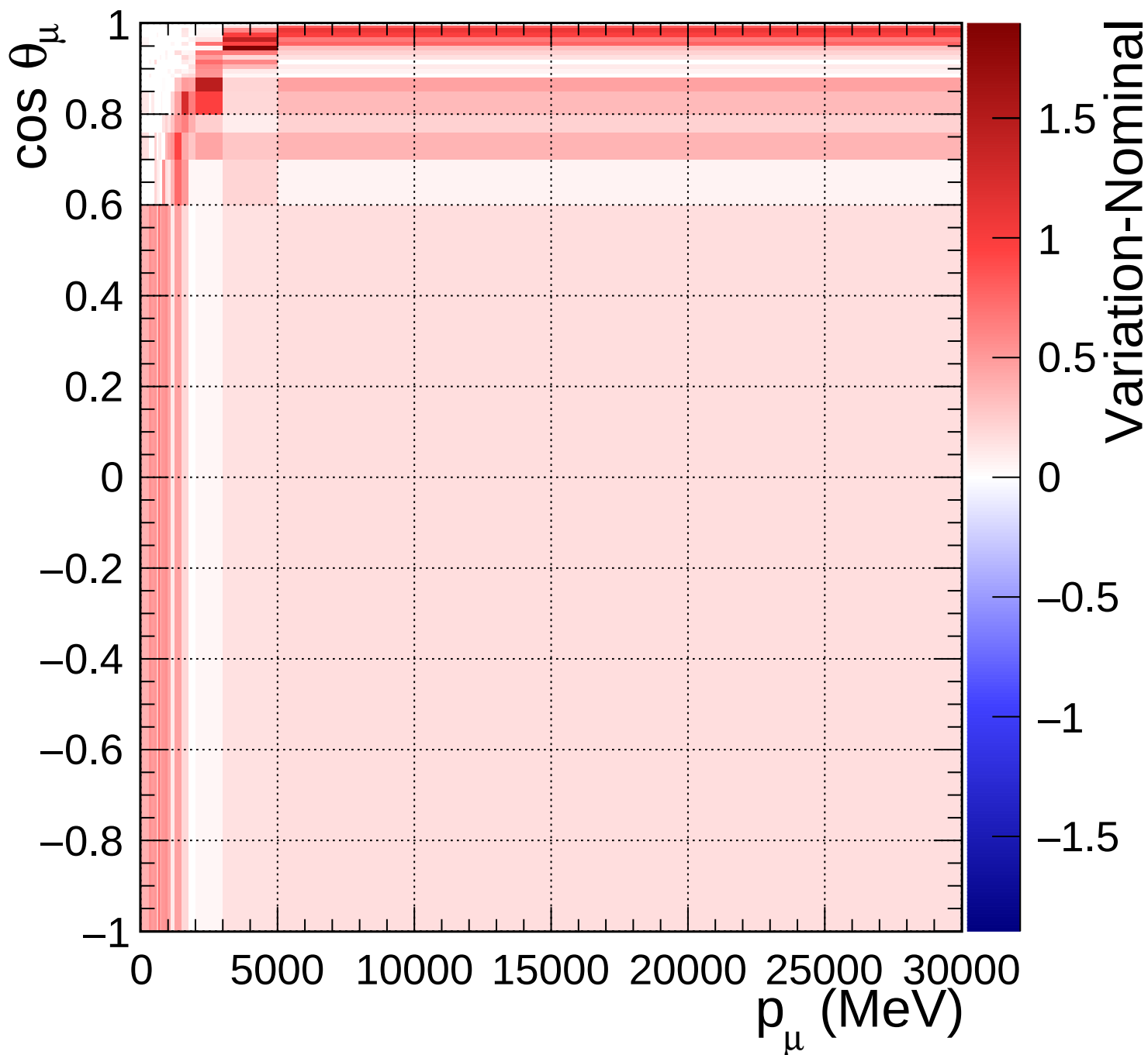
FGD2_numuCC_other_Q2_norm_7_2.2
