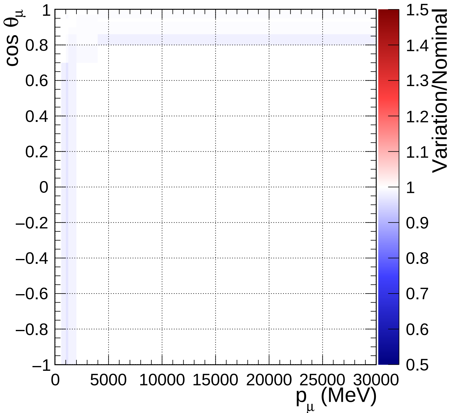
FGD2_NuMuBkg_CCother_in_AntiNu_Mode_Q2_norm_7_0.6
