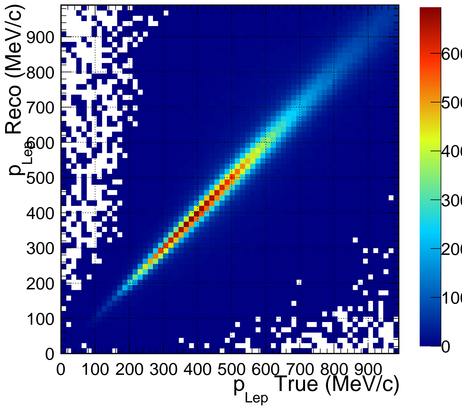
LepCandReco_Mom:LepCandTrue_Mom
