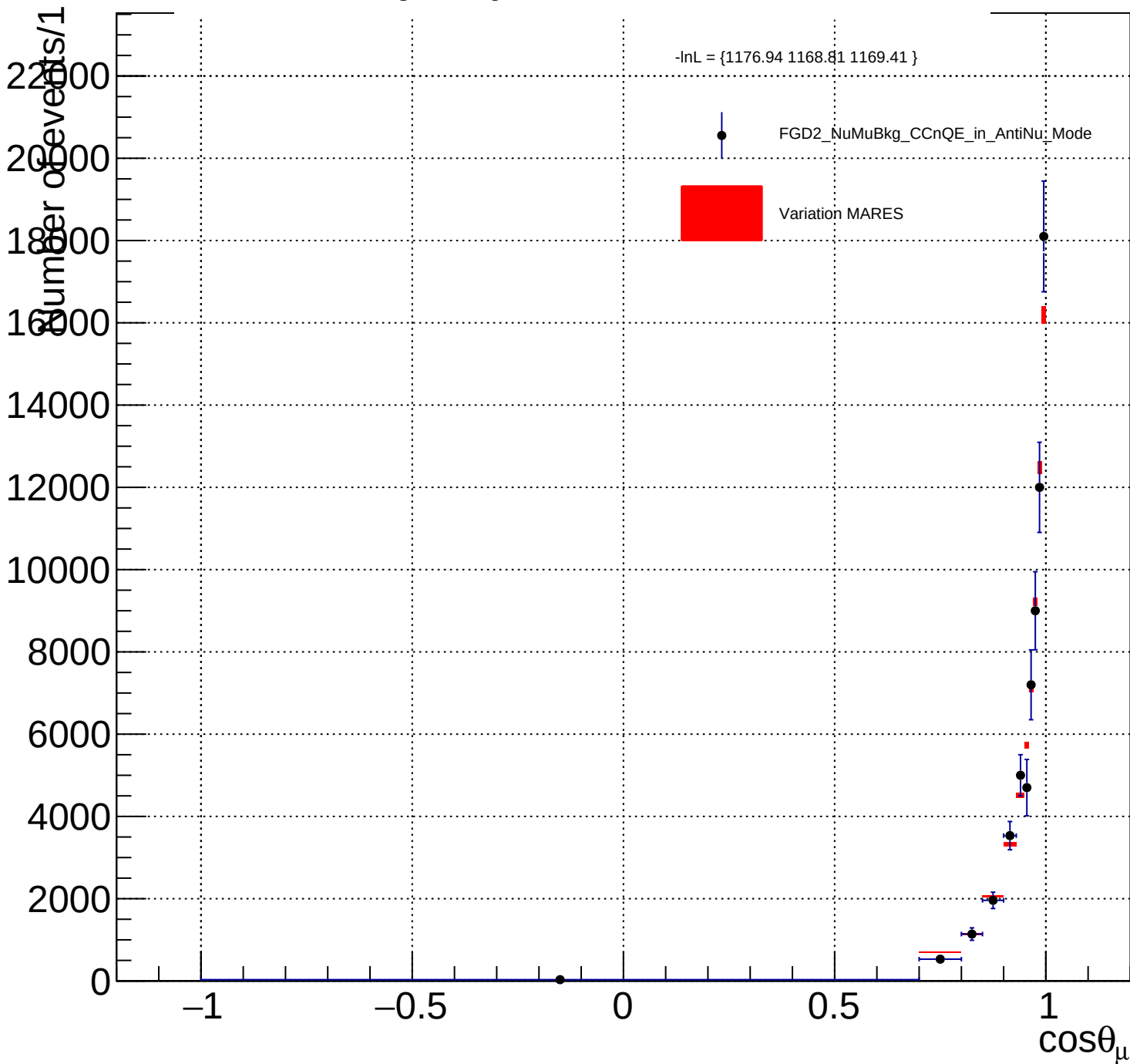
FGD2_NuMuBkg_CCnQE_in_AntiNu_Mode_MARES_Y_norm
