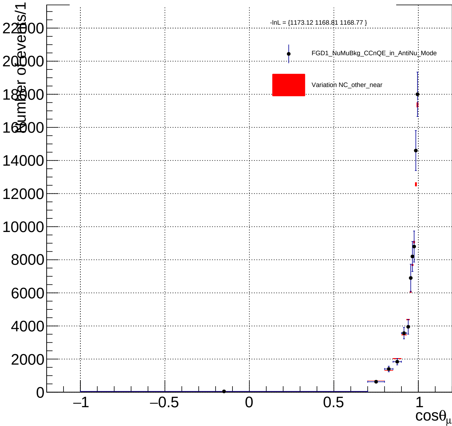
FGD1_NuMuBkg_CCnQE_in_AntiNu_Mode_NC_other_near_Y_norm
