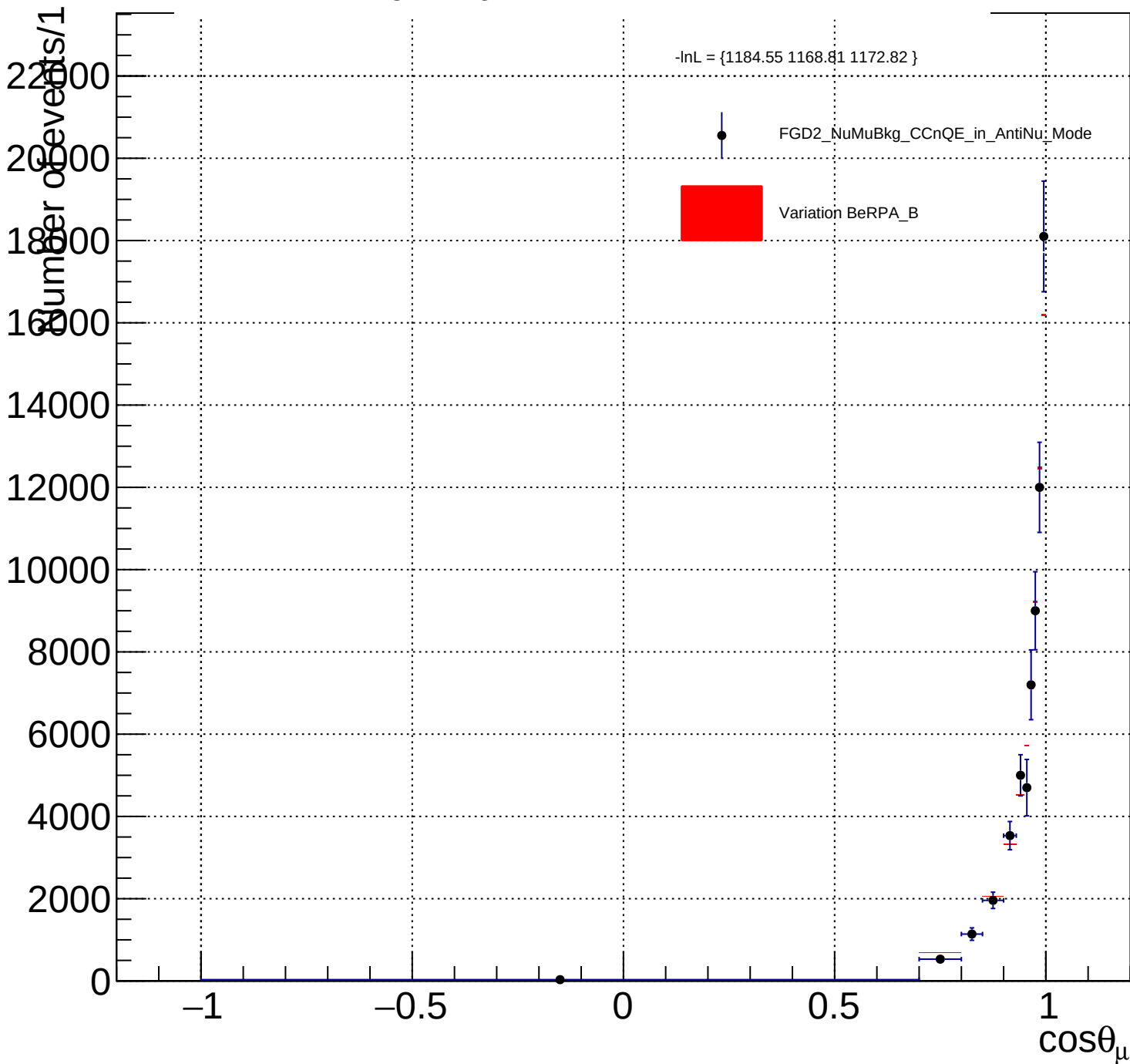
FGD2_NuMuBkg_CCnQE_in_AntiNu_Mode_BeRPA_B_Y_norm
