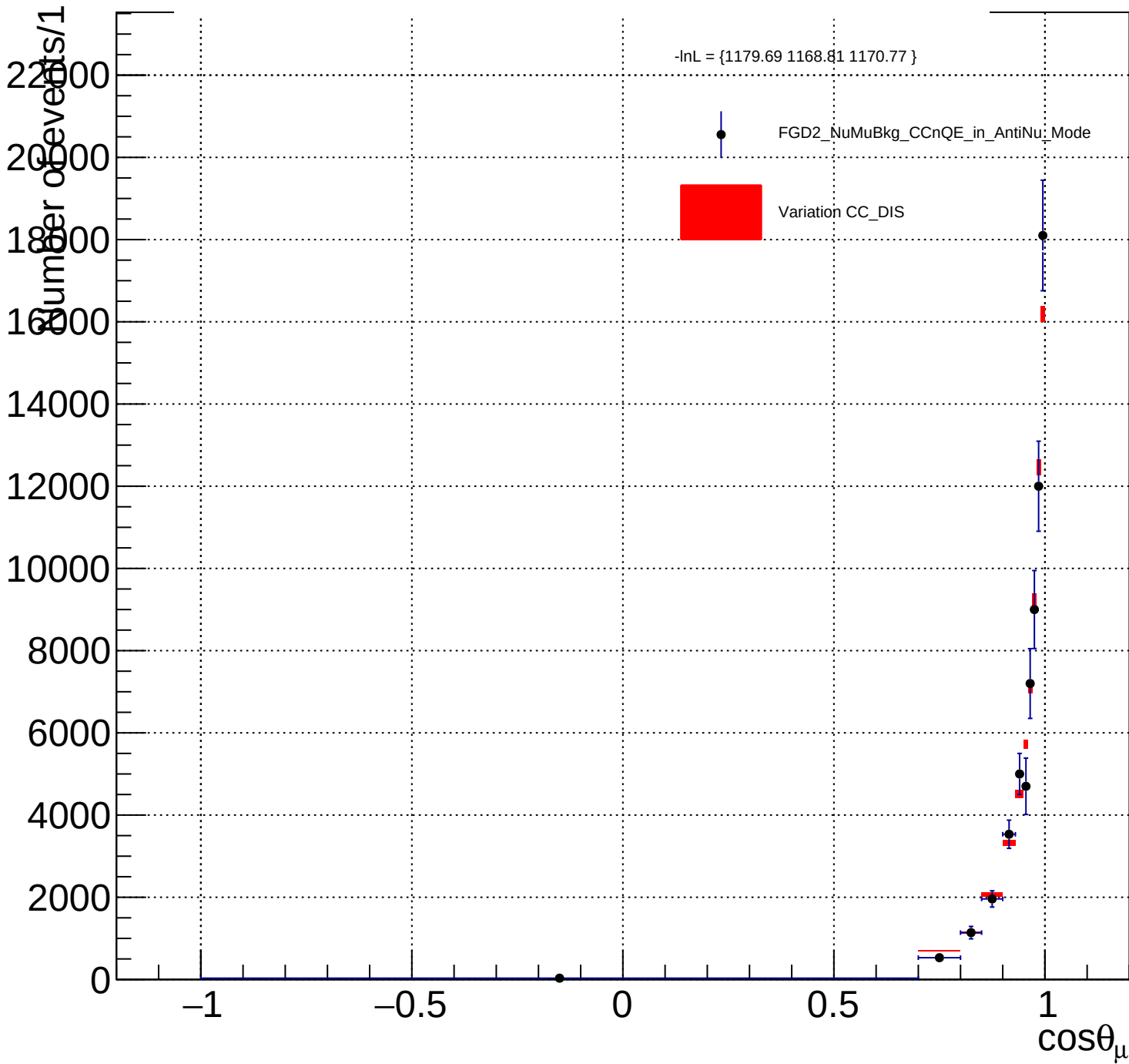
FGD2_NuMuBkg_CCnQE_in_AntiNu_Mode_CC_DIS_Y_norm
