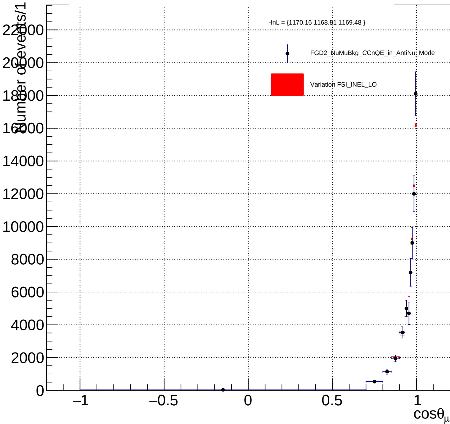
FGD2_NuMuBkg_CCnQE_in_AntiNu_Mode_FSI_INEL_LO_Y_norm
