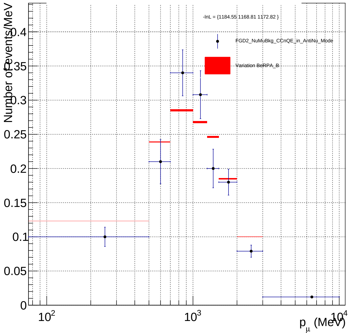
FGD2_NuMuBkg_CCnQE_in_AntiNu_Mode_BeRPA_B_X_norm
