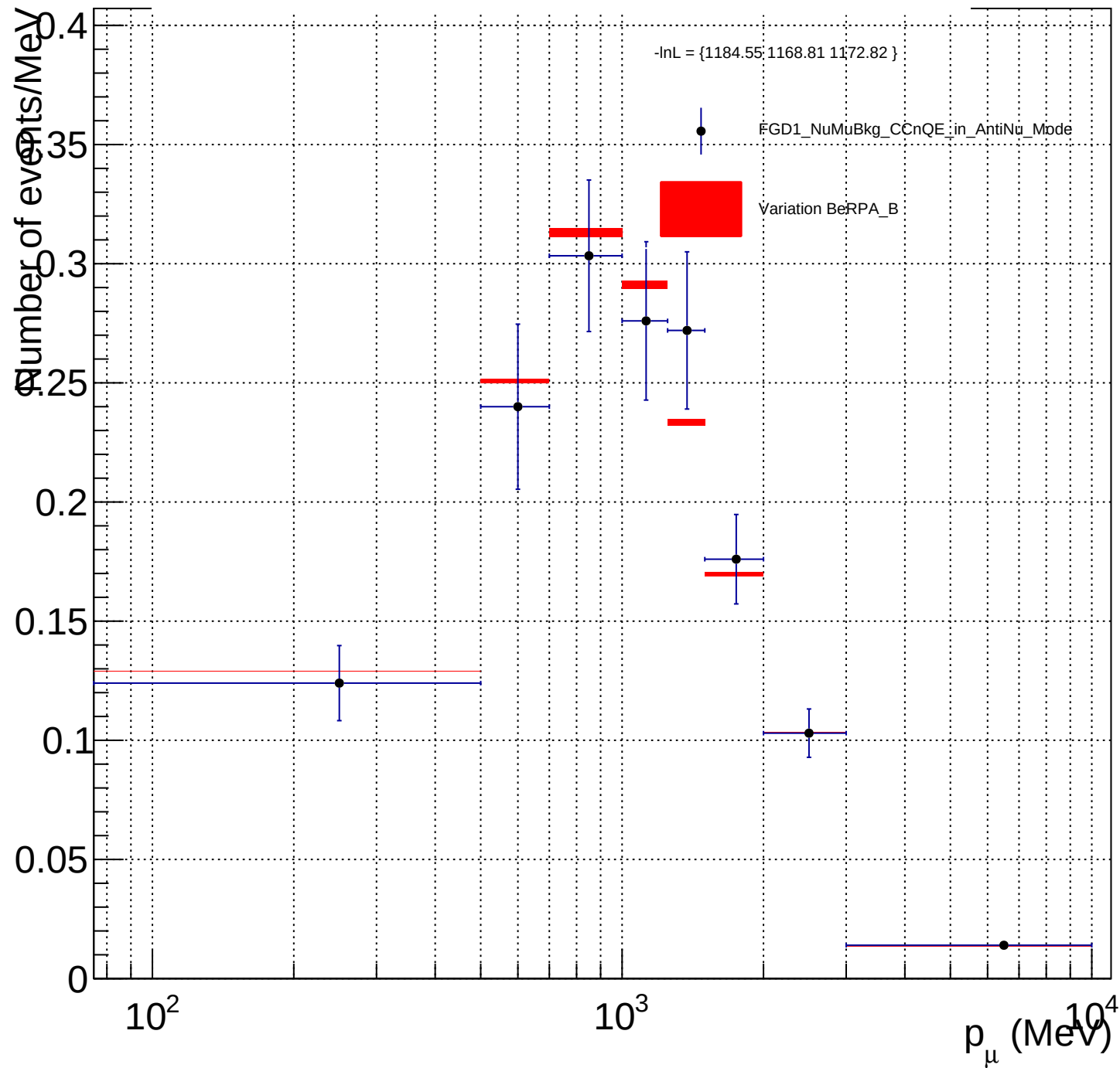
FGD1_NuMuBkg_CCnQE_in_AntiNu_Mode_BeRPA_B_X_norm
