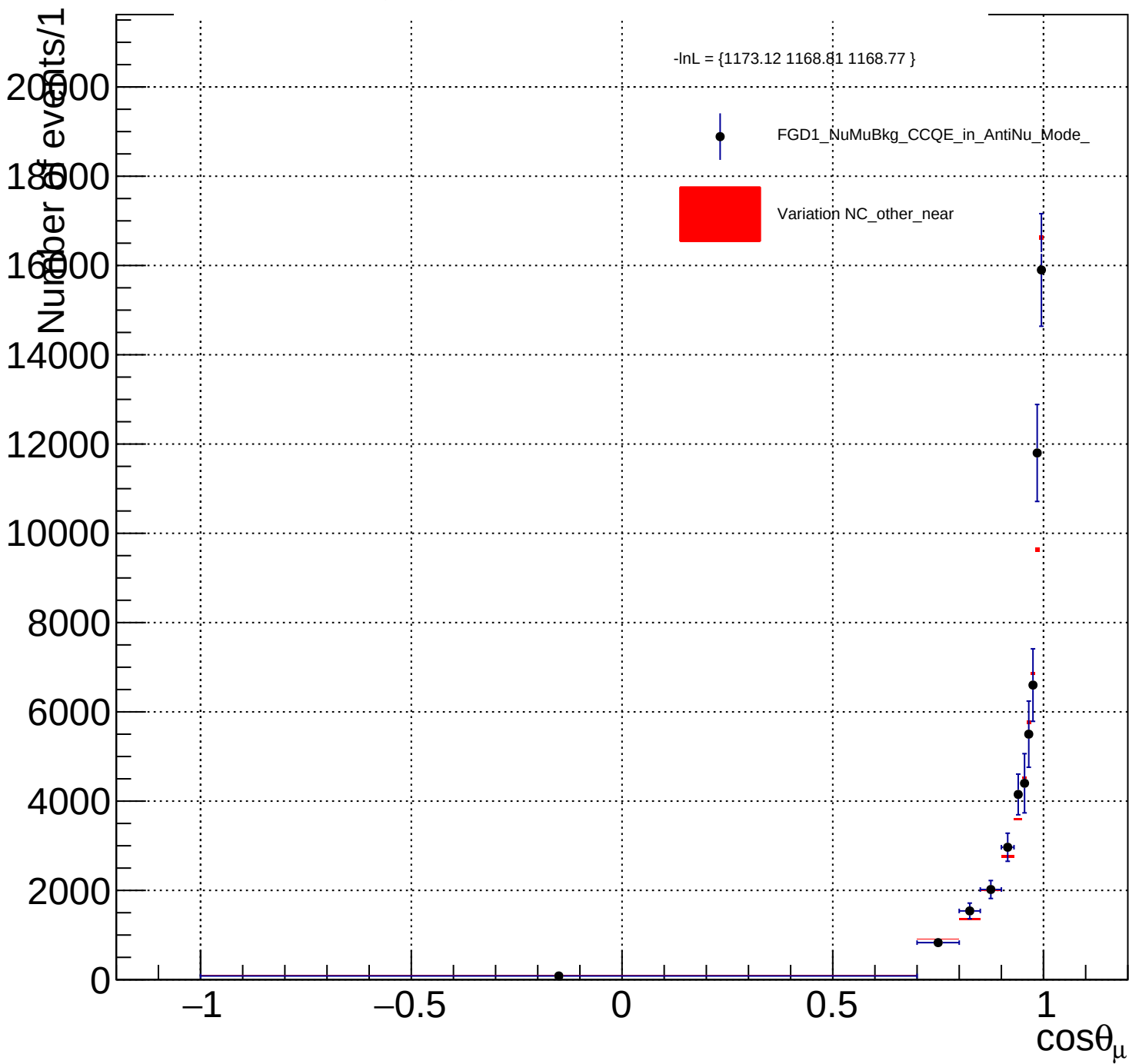
FGD1_NuMuBkg_CCQE_in_AntiNu_Mode_NC_other_near_Y_norm
