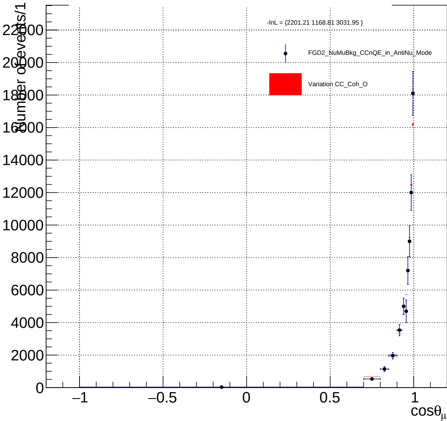
FGD2_NuMuBkg_CCnQE_in_AntiNu_Mode_CC_Coh_O_Y_norm
