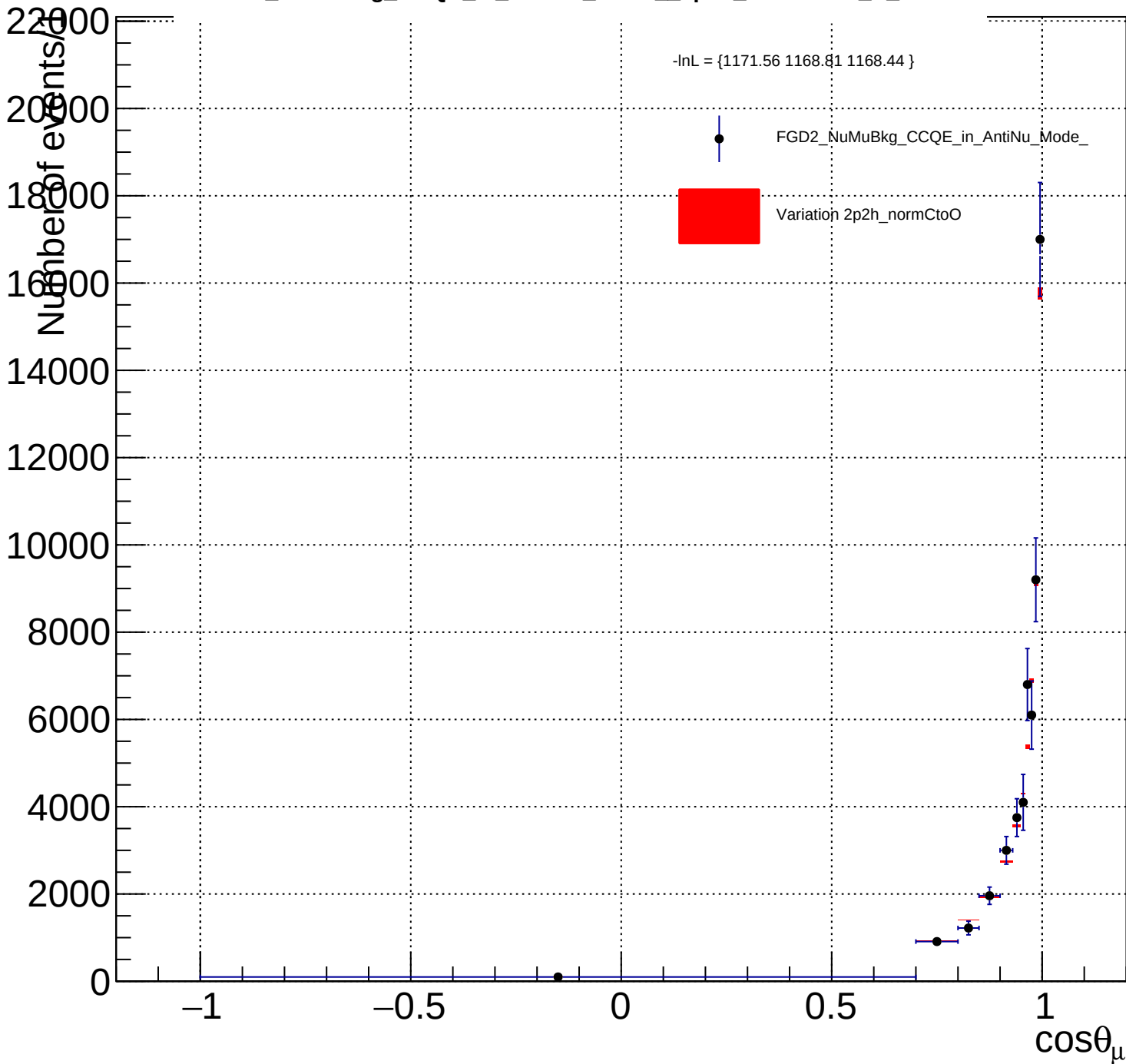
FGD2_NuMuBkg_CCQE_in_AntiNu_Mode_2p2h_normCtoO_Y_norm
