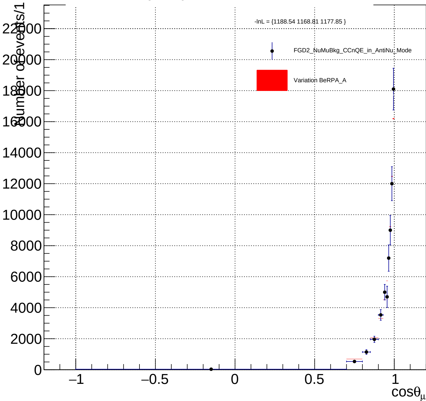
FGD2_NuMuBkg_CCnQE_in_AntiNu_Mode_BeRPA_A_Y_norm
