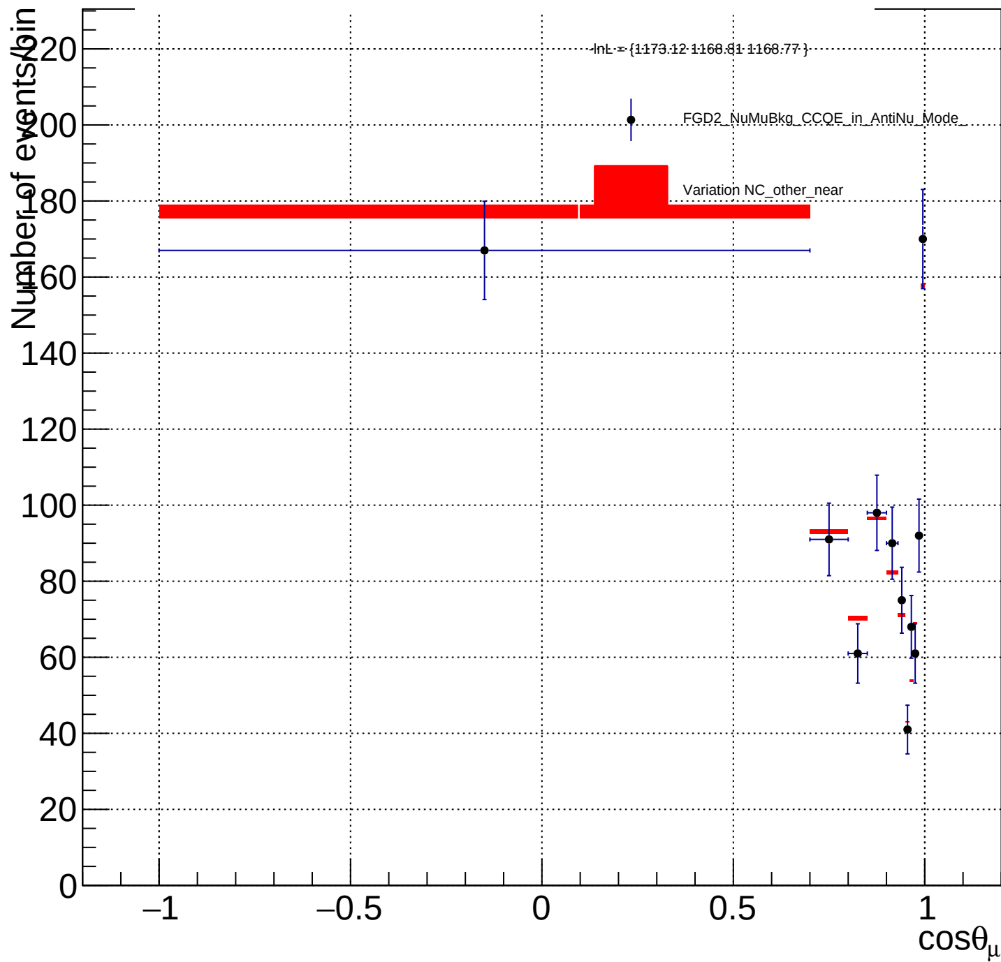
FGD2_NuMuBkg_CCQE_in_AntiNu_Mode__NC_other_near_Y
