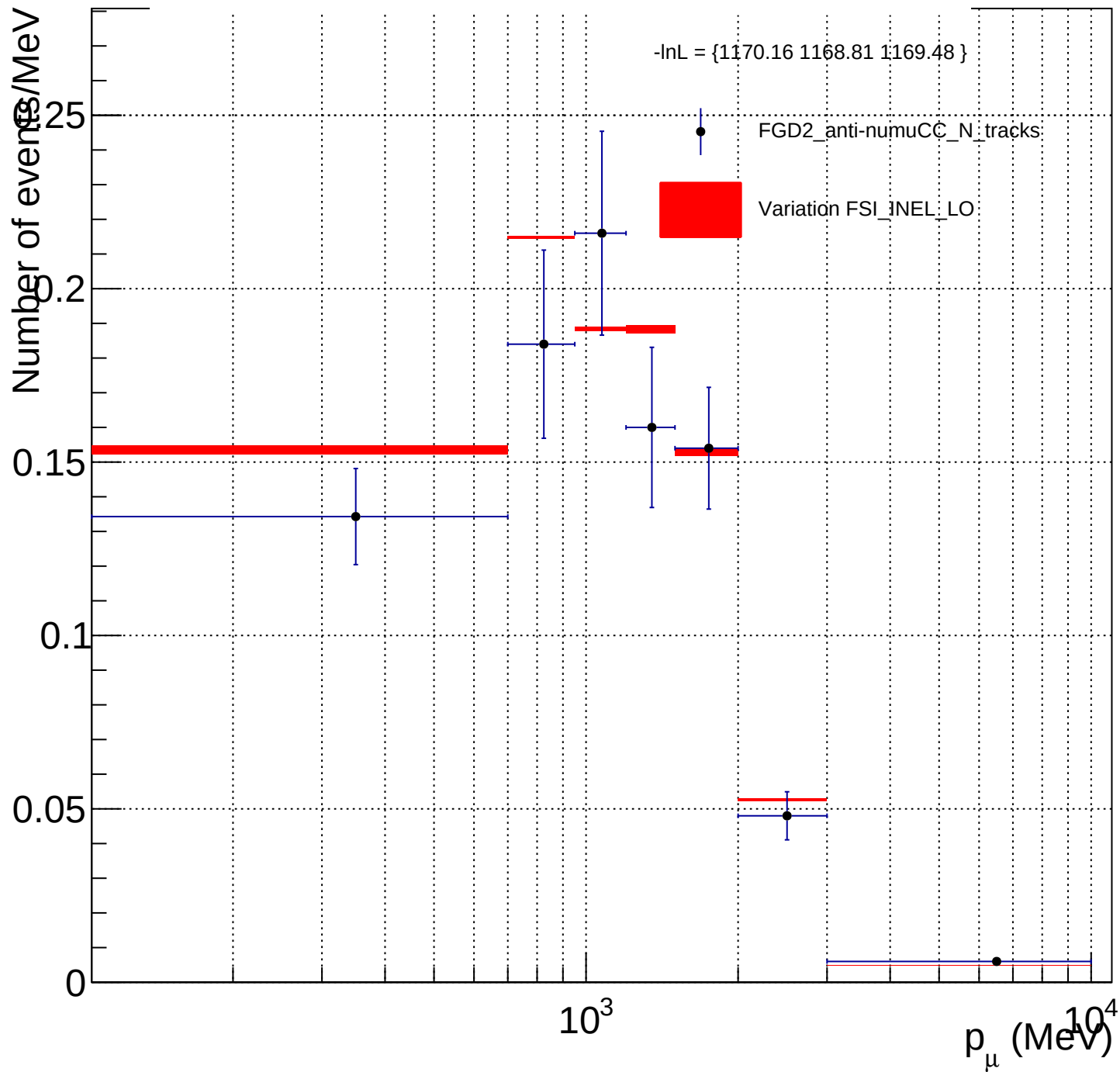
FGD2_anti-numuCC_N_tracks_FSI_INEL_LO_X_norm
