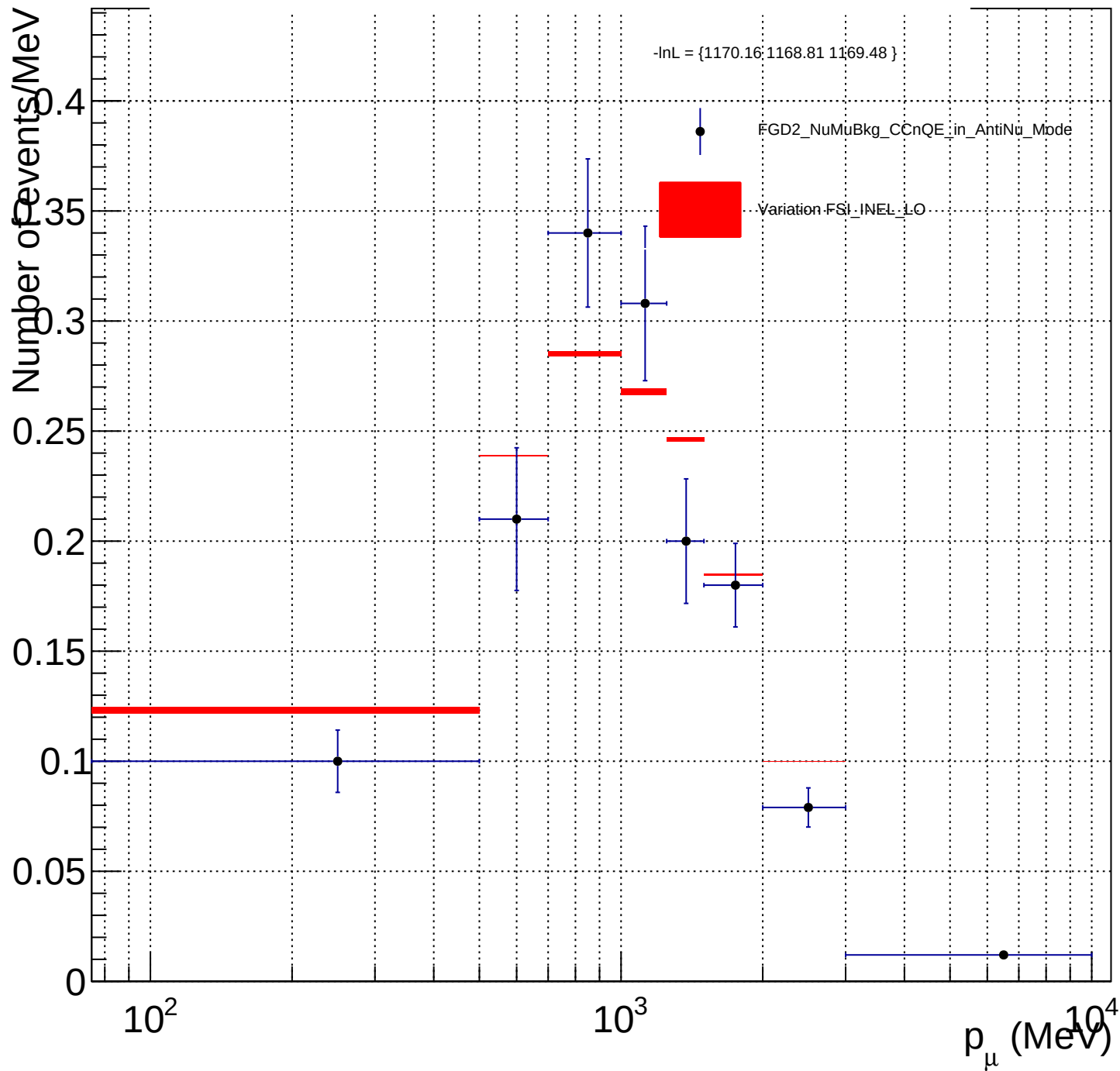
FGD2_NuMuBkg_CCnQE_in_AntiNu_Mode_FSI_INEL_LO_X_norm
