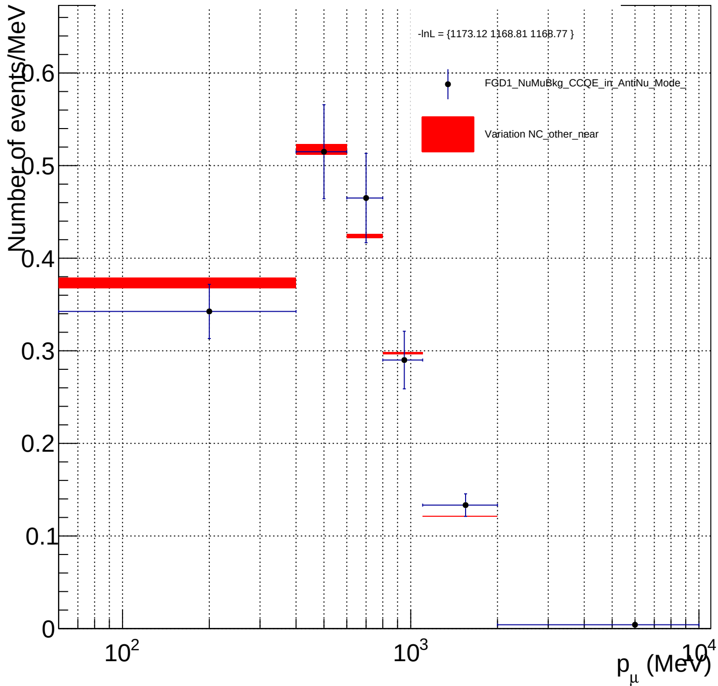
FGD1_NuMuBkg_CCQE_in_AntiNu_Mode_NC_other_near_X_norm
