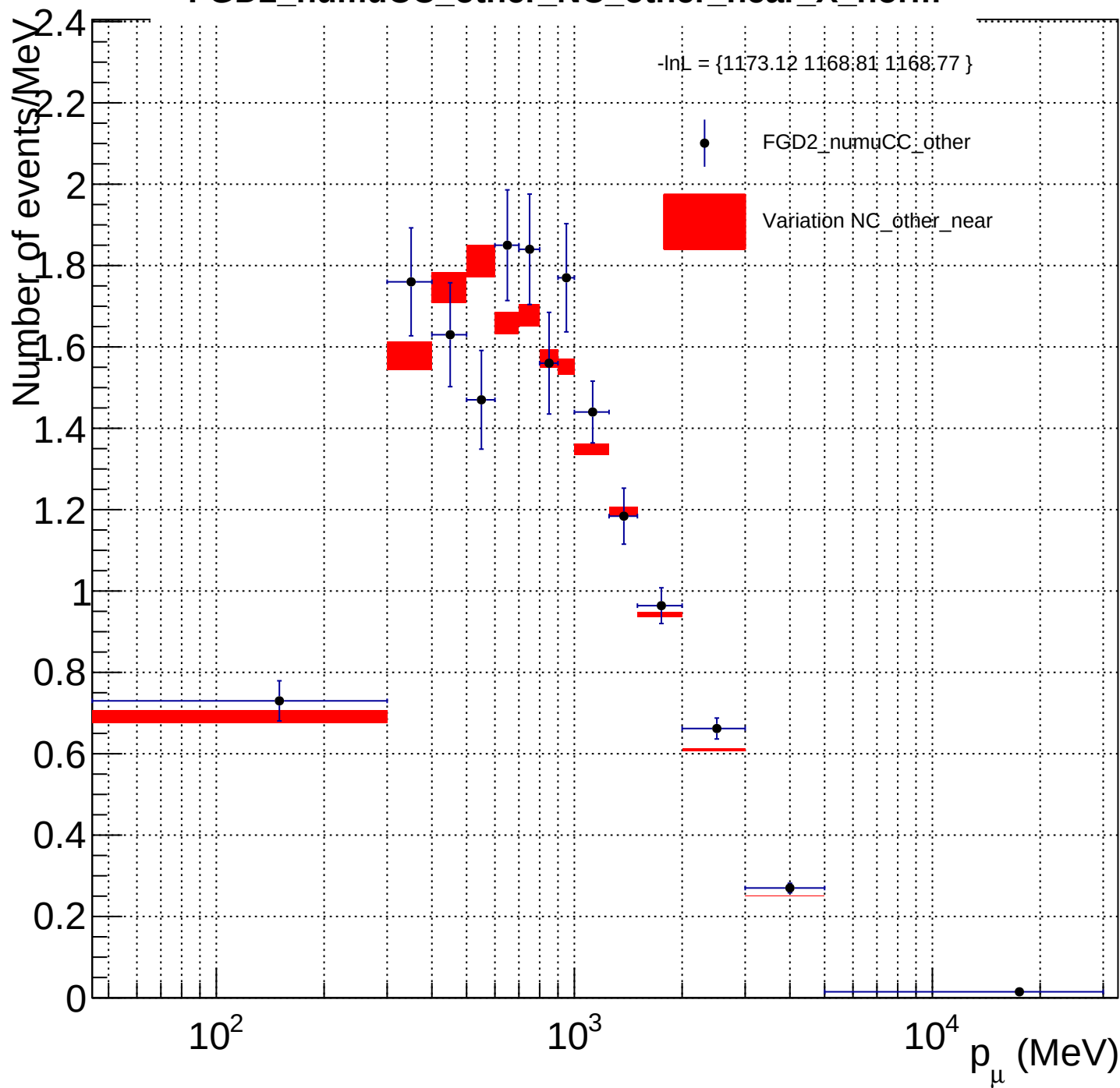
FGD2_numuCC_other_NC_other_near_X_norm
