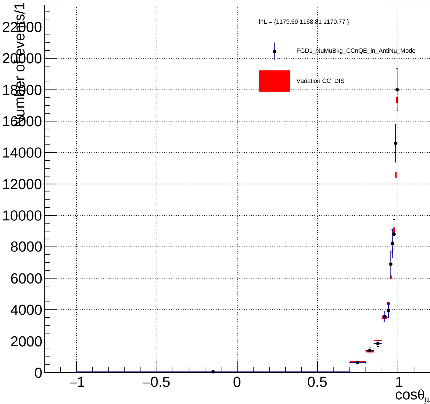
FGD1_NuMuBkg_CCnQE_in_AntiNu_Mode_CC_DIS_Y_norm
