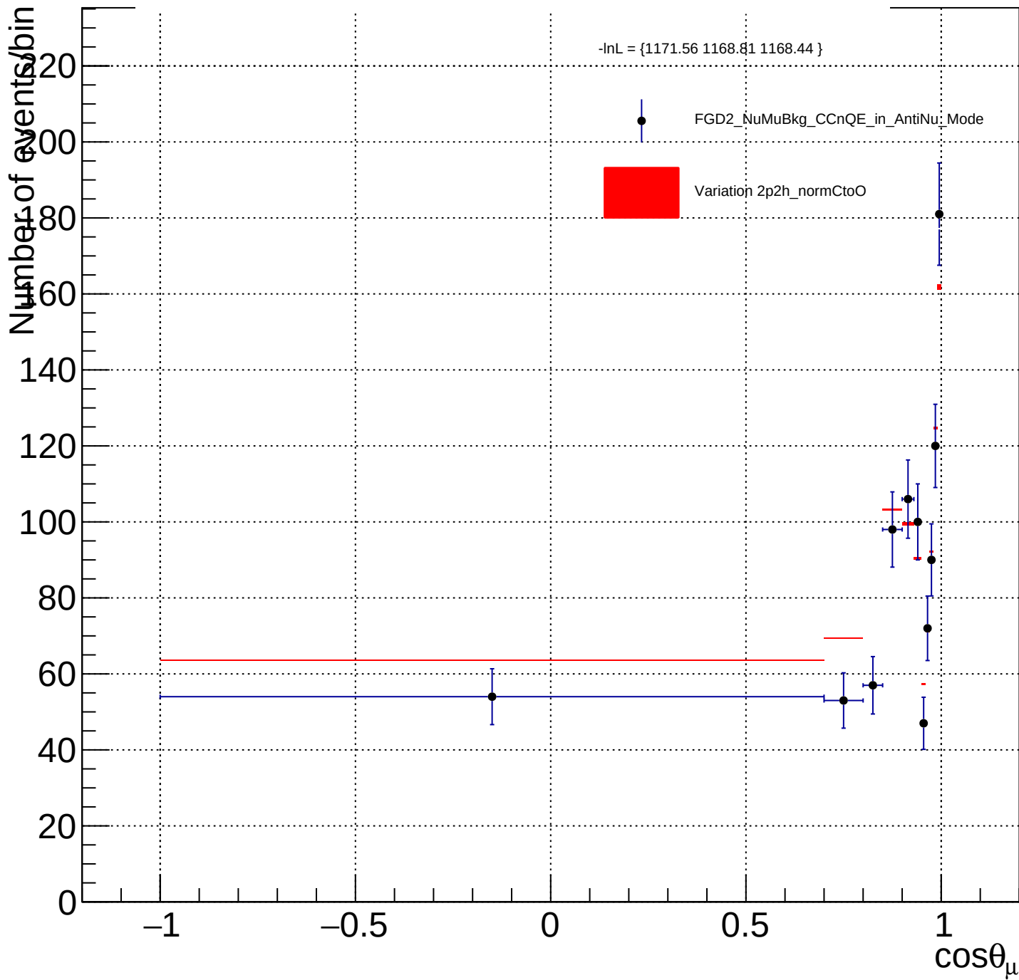
FGD2_NuMuBkg_CCnQE_in_AntiNu_Mode_2p2h_normCtoO_Y
