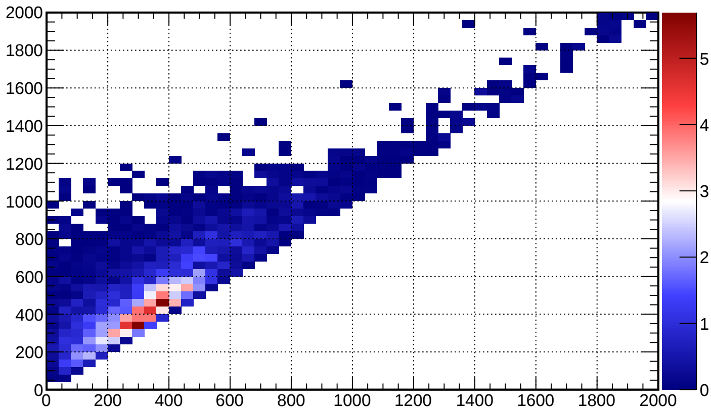
FGD1_anti-numuCC_QE_2p2h_shape_C_nubar_1_2p2h
